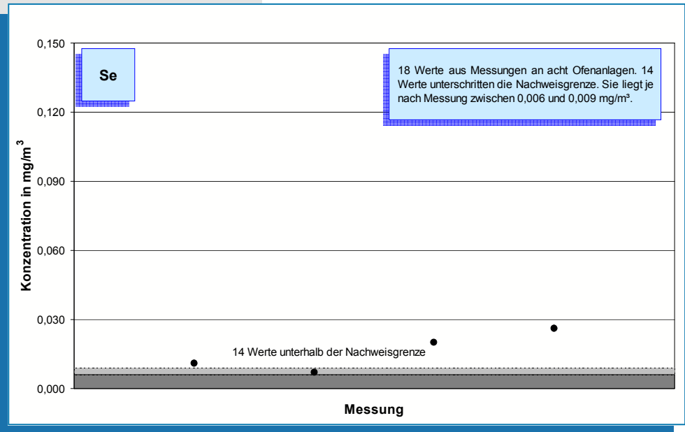
Bild 5-53: Messwerte (Jahr 2006) der Selen-Konzentration im Reingas von acht Drehofenanlagen.
