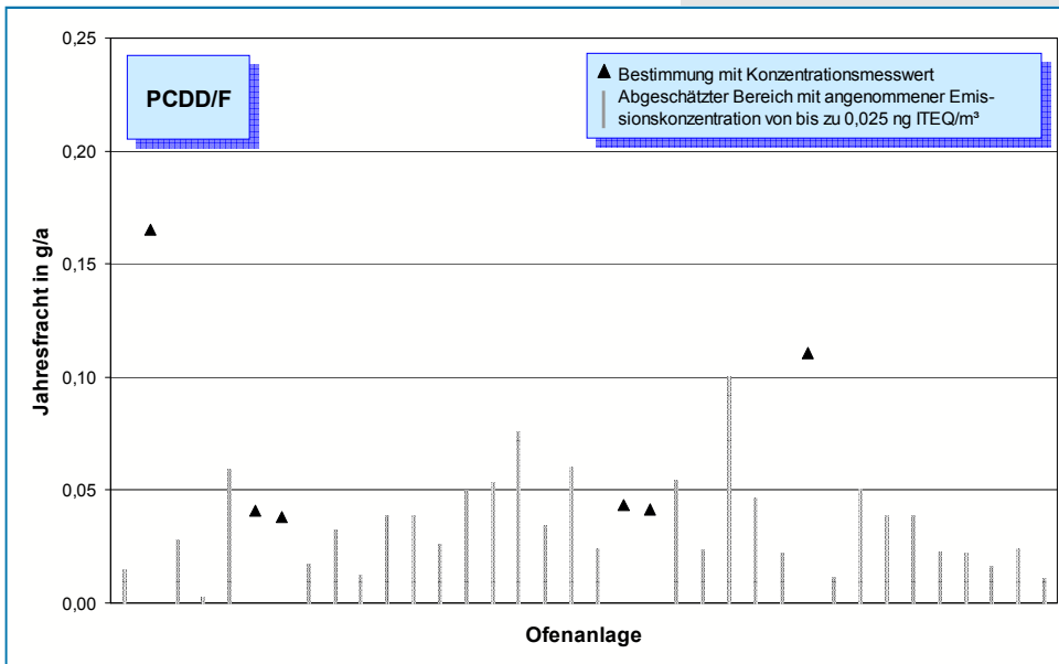
Bild 5-12: Dioxin- und Furan-Emissionen (Jahresfracht 2006) von 36 Drehofenanlagen.
