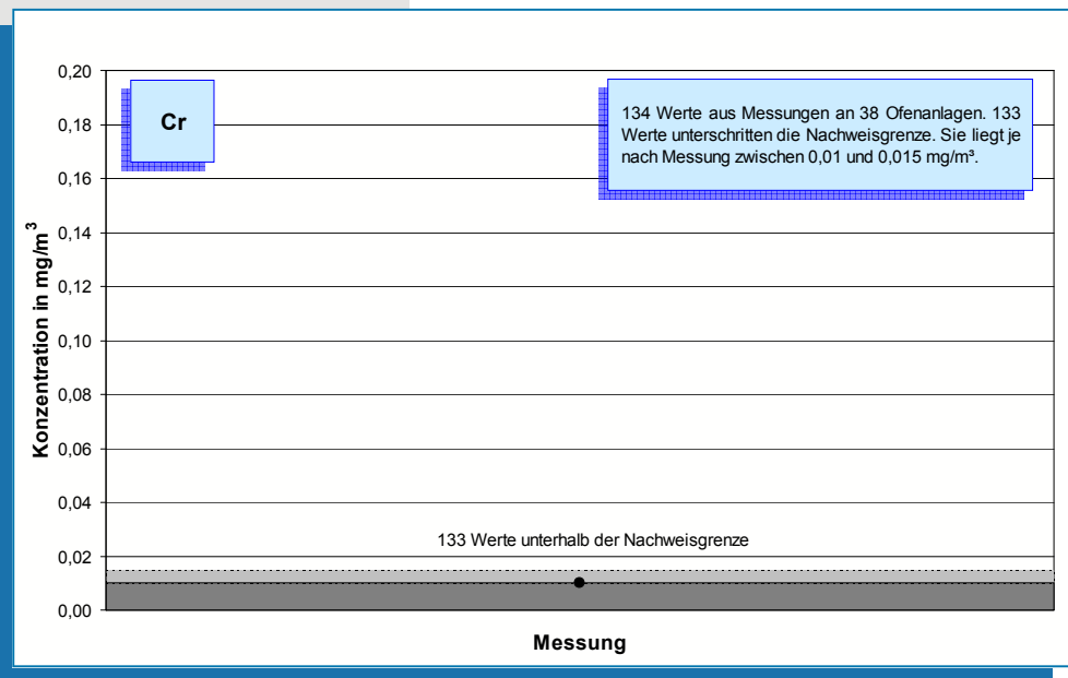
Bild 5-37: Messwerte (Jahr 2006) der Chrom-Konzentration im Reingas von 38 Drehofenanlagen.
