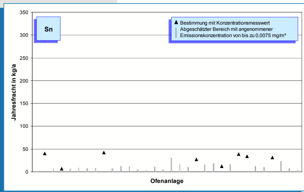
Bild 5-50: Zinn-Emissionen (Jahresfracht 2006) von 32 Drehofenanlagen. Bei Messungen unterhalb der Nachweisgrenze kann die Fracht nur abgeschätzt werden. Der Bereich möglicher Emissionen ist in diesen Fällen als Linie dargestellt, deren Obergrenze mit einer Konzentration von 0,0075 mg/m 3 berechnet wurde.
