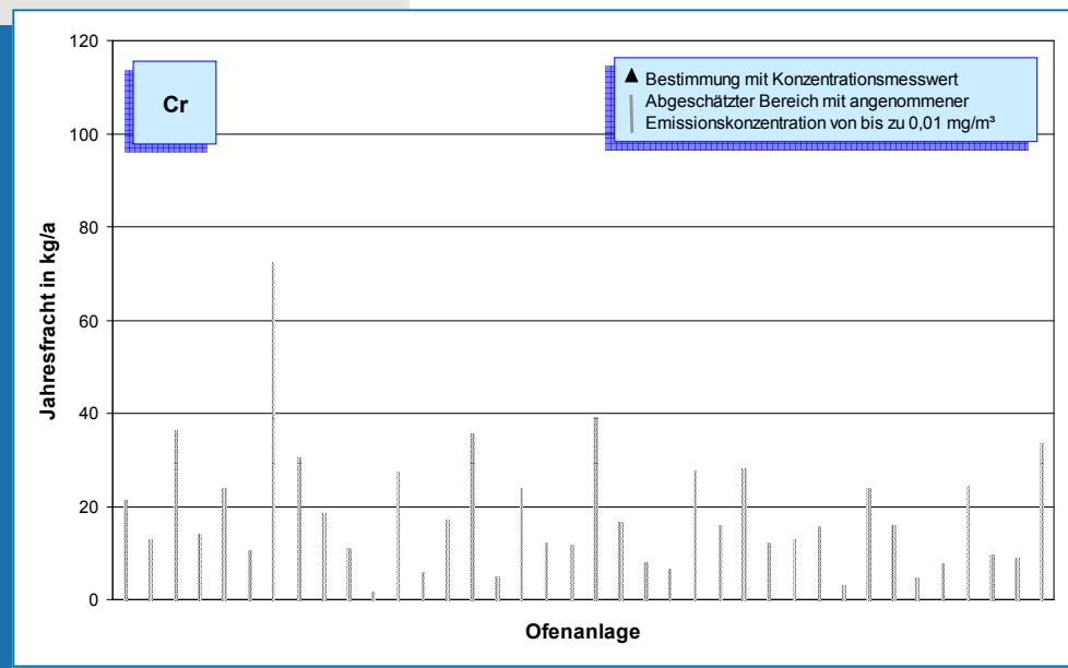
Bild 5-38: Chrom-Emissionen (Jahresfracht 2006) von 38 Drehofenanlagen. Bei Messungen unterhalb der Nachweisgrenze kann die Fracht nur abgeschätzt werden. Der Bereich möglicher Emissionen ist in diesen Fällen als Linie dargestellt, deren Obergrenze mit einer Konzentration von 0,01 mg/m 3 berechnet wurde.
