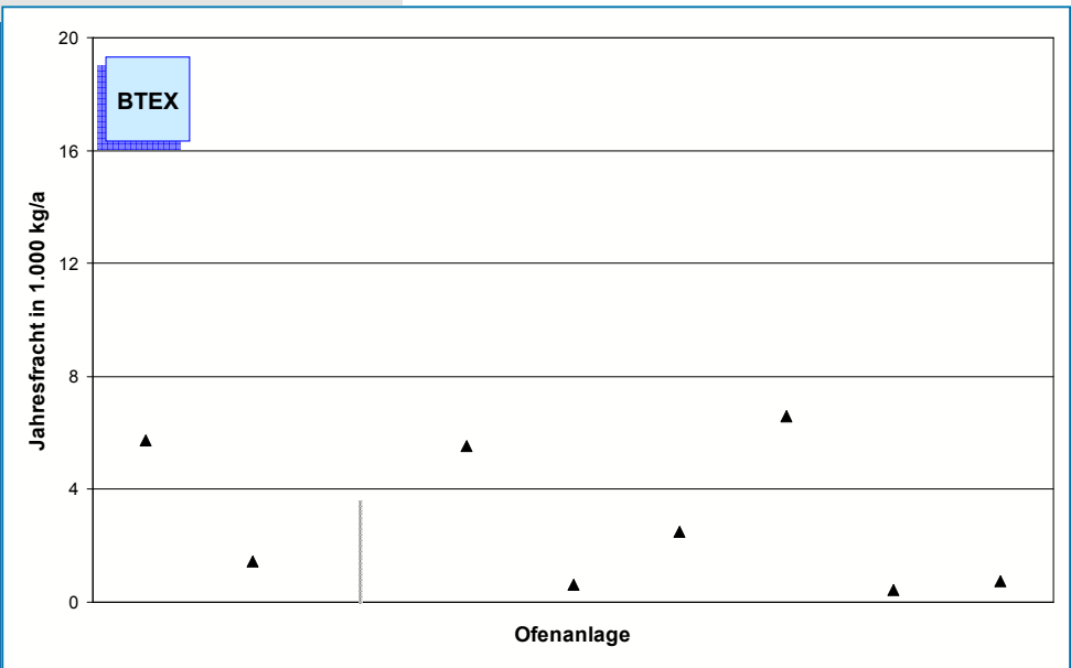
Bild 5-18: BTEX-Emissionen (Jahresfracht 2006) von neun Drehofenanlagen.
