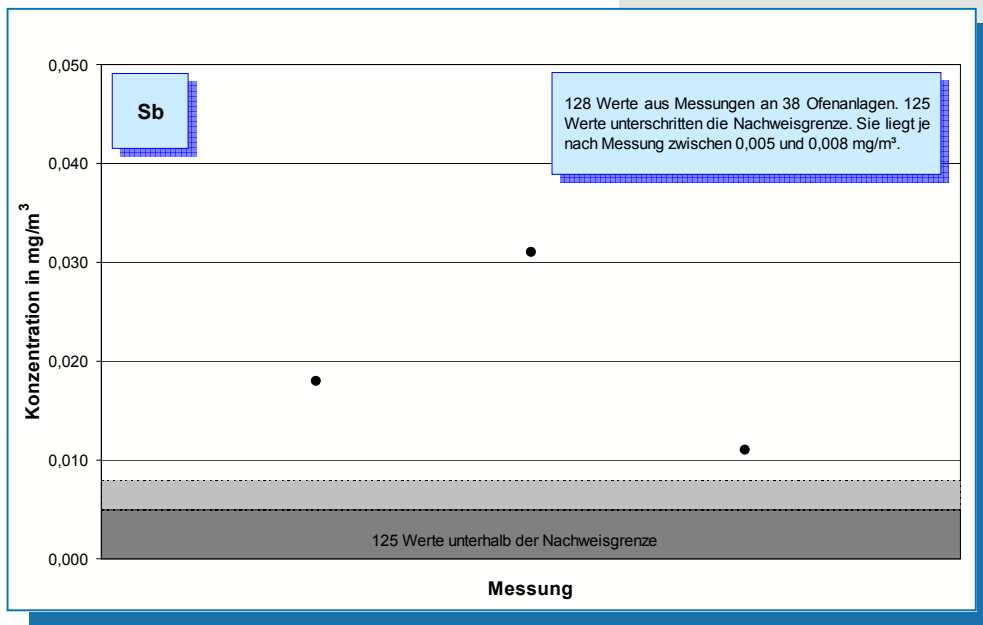
Bild 5-31: Messwerte (Jahr 2006) der Antimon-Konzentration im Reingas von 38 Drehofenanlagen.
