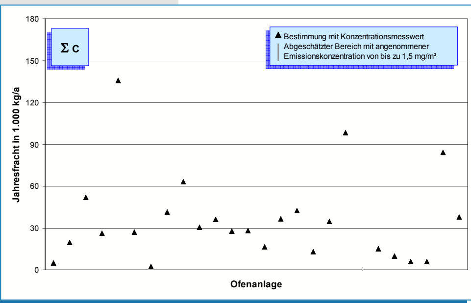
Bild 5-10: Emissionen von organischem Gesamtkohlenstoff (Jahresfracht 2006) von 26 Drehofenanlagen.
