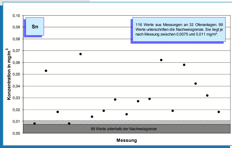
Bild 5-49: Messwerte (Jahr 2006) der Zinn-Konzentration im Reingas von 32 Drehofenanlagen.
