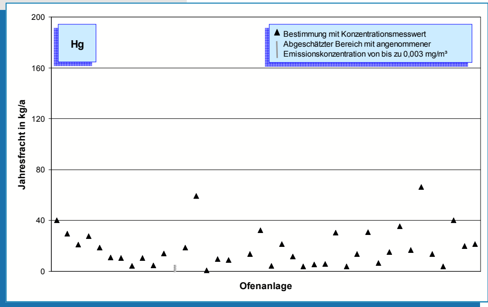
Bild 5-30: Quecksilber-Emissionen (Jahresfracht 2006) von 40 Drehofenanlagen. Bei Messungen unterhalb der Nachweisgrenze kann die Fracht nur abgeschätzt werden. Der Bereich möglicher Emissionen ist in diesen Fällen als Linie dargestellt, deren Obergrenze mit einer Konzentration von 0,003 mg/m 3 berechnet wurde.
