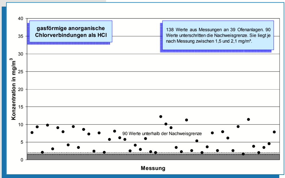
Bild 5-21: Messwerte (Jahr 2006) der Konzentrationen gasförmiger anorganischer Chlorverbindungen, berechnet als HCl, im Reingas von 39 Drehofenanlagen.
