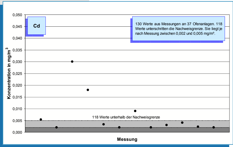
Bild 5-25: Messwerte (Jahr 2006) der Cadmium-Konzentration im Reingas von 37 Drehofenanlagen.
