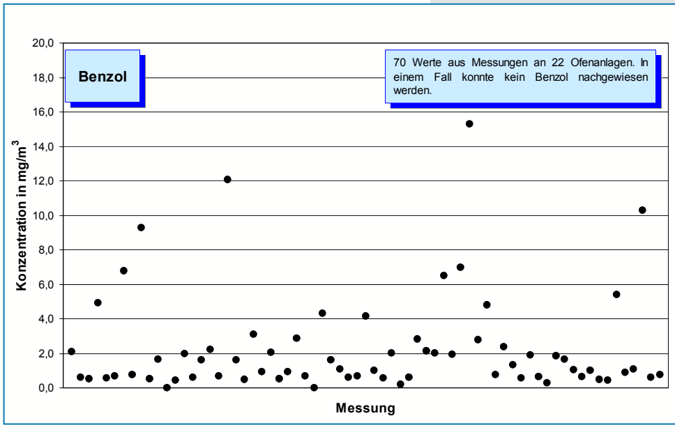
Bild 5-19: Messwerte (Jahr 2006) der Konzentration von Benzol im Reingas von 22 Drehofenanlagen. In einem Fall konnte kein Benzol nachgewiesen werden. Eine Nachweisgrenze lässt sich aus der Norm nicht ableiten. Bei den derzeit eingesetzten Messverfahren sind gemessene Emissionskonzentrationen unterhalb von 0,013 mg/m 3 nicht abgesichert.
