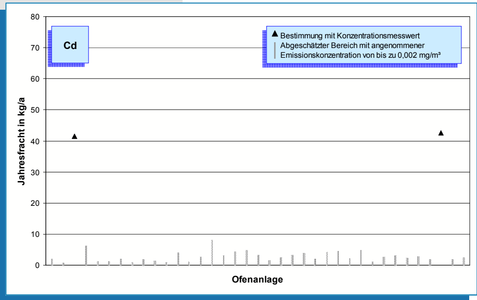
Bild 5-26: Cadmium-Emissionen (Jahresfracht 2006) von 37 Drehofenanlagen. Bei Messungen unterhalb der Nachweisgrenze kann die Fracht nur abgeschätzt werden. Der Bereich möglicher Emissionen ist in diesen Fällen als Linie dargestellt, deren Obergrenze mit einer Konzentration von 0,002 mg/m 3 berechnet wurde.
