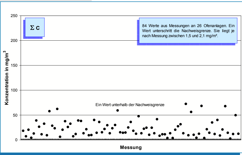
Bild 5-9: Messwerte (Jahr 2006) der Konzentration von organischem Gesamtkohlenstoff im Reingas von 26 Drehofenanlagen.
