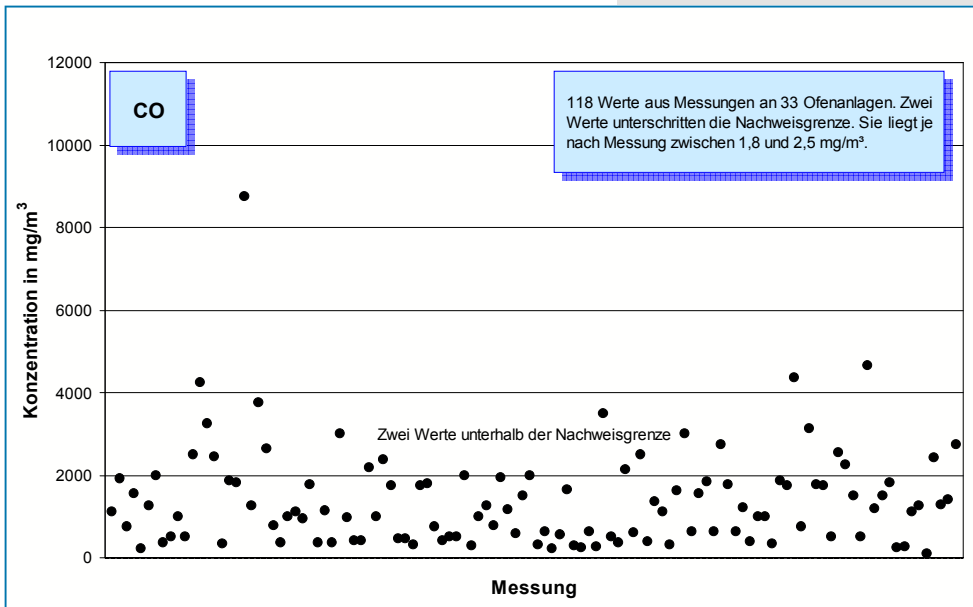
Bild 5-7: Messwerte (Jahr 2006) der CO-Konzentration im Reingas von 33 Drehofenanlagen. In zwei Fällen konnte kein CO nachgewiesen werden.
