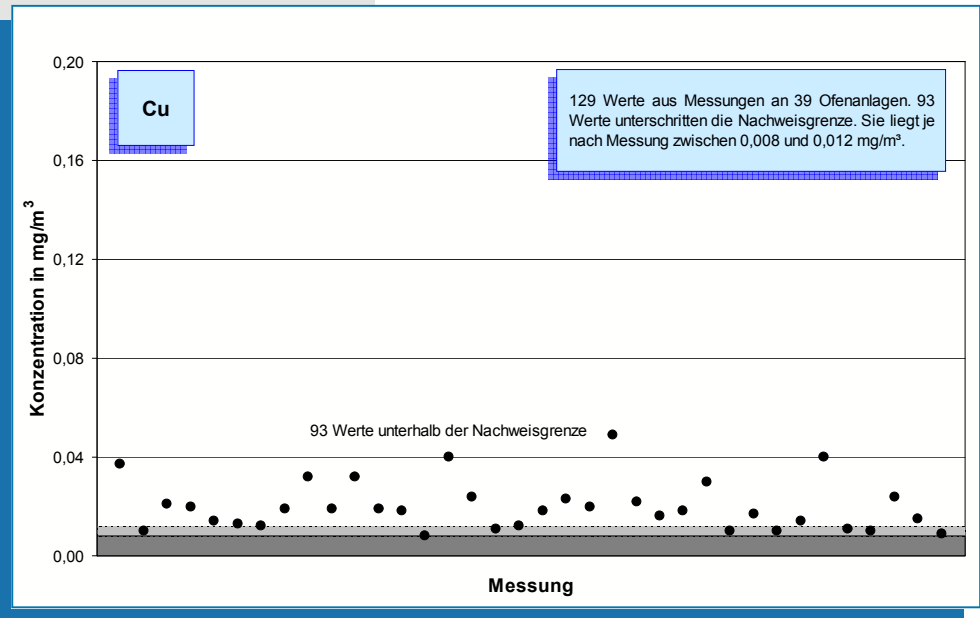
Bild 5-41: Messwerte (Jahr 2006) der Kupfer-Konzentration im Reingas von 39 Drehofenanlagen.
