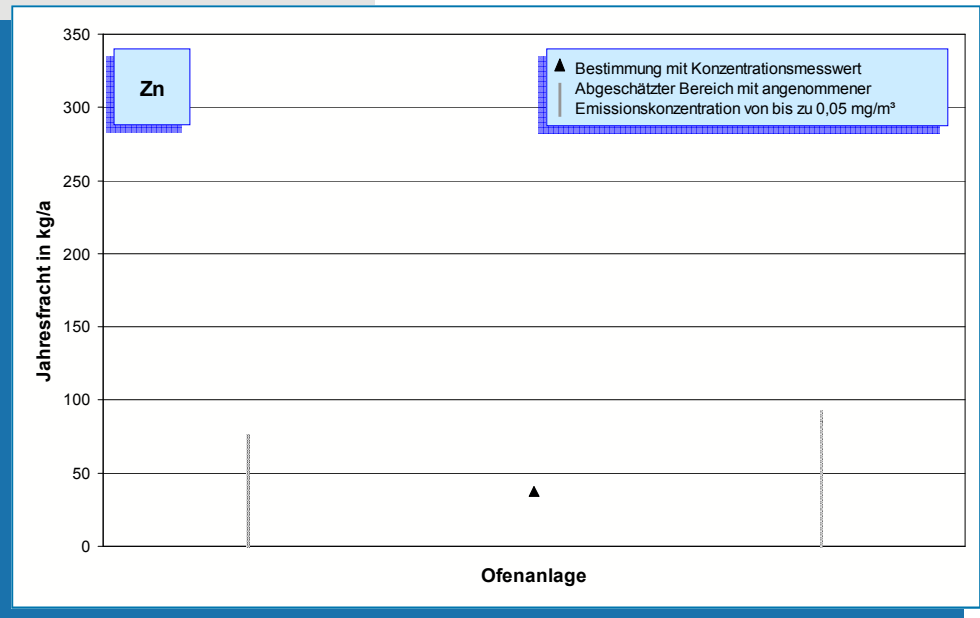
Bild 5-58: Zink-Emissionen (Jahresfracht 2006) von drei Drehofenanlagen.
