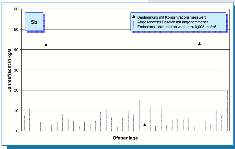
Bild 5-32: Antimon-Emissionen (Jahresfracht 2006) von 38 Drehofenanlagen.
