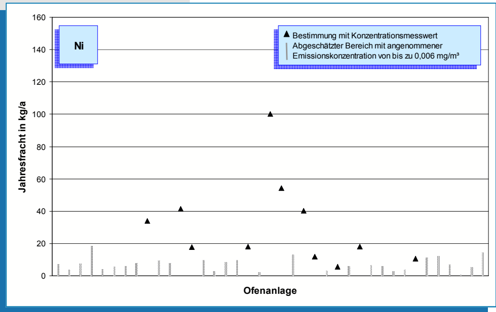
Bild 5-46: Nickel-Emissionen (Jahresfracht 2006) von 39 Drehofenanlagen. Bei Messungen unterhalb der Nachweisgrenze kann die Fracht nur abgeschätzt werden. Der Bereich möglicher Emissionen ist in diesen Fällen als Linie dargestellt, deren Obergrenze mit einer Konzentration von 0,006 mg/m 3 berechnet wurde.
