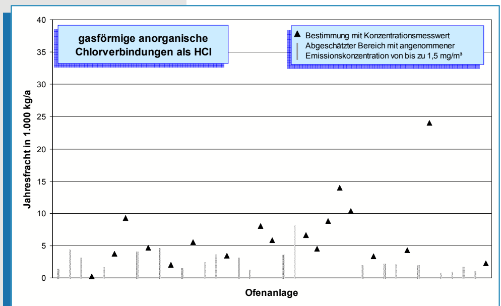
Bild 5-22: HCl-Emissionen (Jahresfracht 2006) von 39 Drehofenanlagen.
