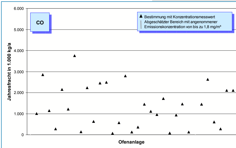
Bild 5-8: CO-Emissionen (Jahresfracht 2006) von 33 Drehofenanlagen.
