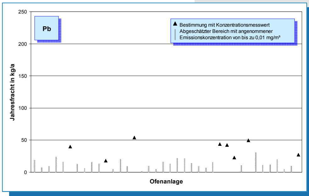
Bild 5-36: Blei-Emissionen (Jahresfracht 2006) von 38 Drehofenanlagen.
