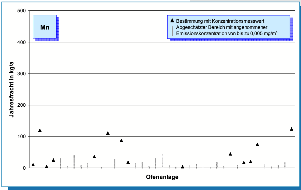
Bild 5-44: Mangan-Emissionen (Jahresfracht 2006) von 39 Drehofenanlagen.
