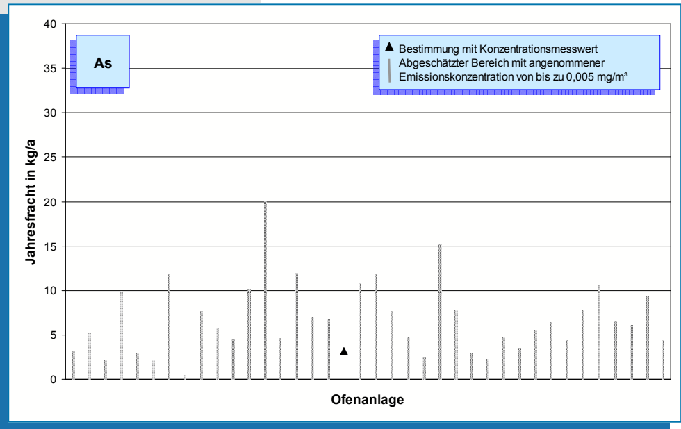
Bild 5-34: Arsen-Emissionen (Jahresfracht 2006) von 38 Drehofenanlagen. Bei Messungen unterhalb der Nachweisgrenze kann die Fracht nur abgeschätzt werden. Der Bereich möglicher Emissionen ist in diesen Fällen als Linie dargestellt, deren Obergrenze mit einer Konzentration von 0,005 mg/m 3 berechnet wurde.
