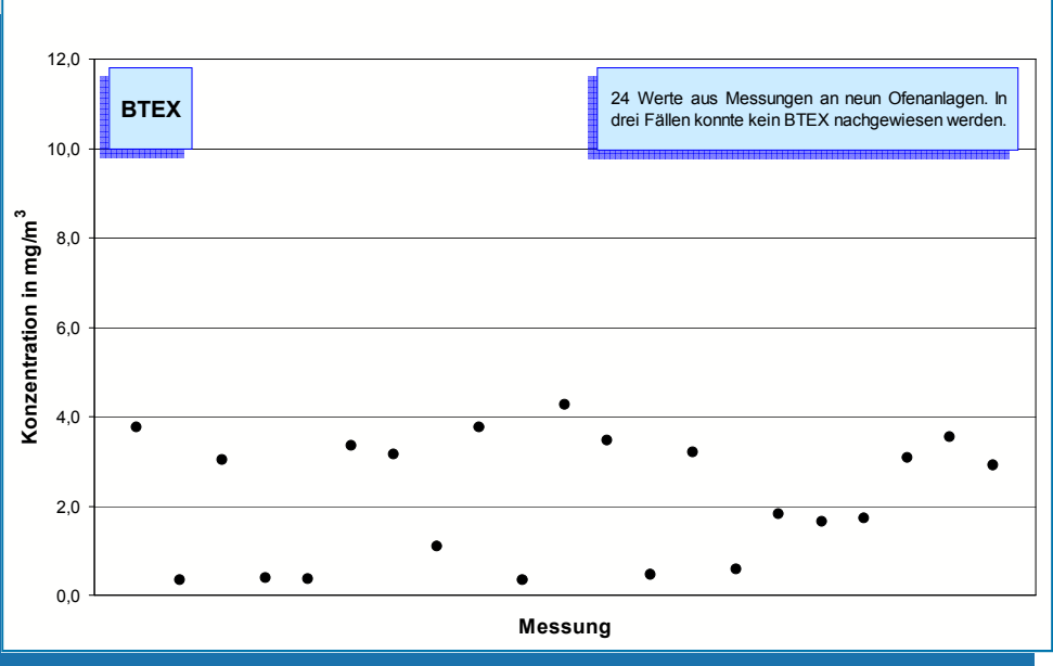
Bild 5-17: Messwerte (Jahr 2006) der Konzentration von BTEX im Reingas von neun Drehofenanlagen. In drei Fällen konnte kein BTEX nachgewiesen werden. Eine Nachweisgrenze lässt sich aus der Norm nicht ableiten. Bei den eingesetzten Messverfahren sind gemessene Emissionskonzentrationen unterhalb von 0,013 mg/m 3 nicht abgesichert.
