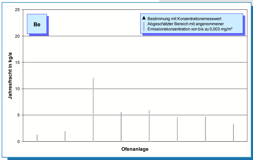
Bild 5-52: Beryllium-Emissionen (Jahresfracht 2006) von acht Drehofenanlagen.
