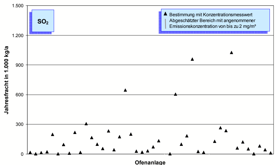
Bild 5-6: SO 2 -Emissionen (Jahresfracht 2006) von 44 Drehofenanlagen. Bei Messungen unterhalb der Nachweisgrenze kann die Fracht nur abgeschätzt werden. Der Bereich möglicher Emissionen ist in diesen Fällen als Linie dargestellt, deren Obergrenze mit einer Konzentration von 2 mg/m 3 berechnet wurde.
