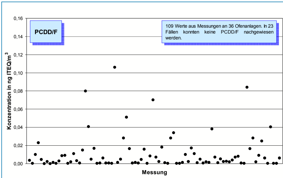
Bild 5-11: Messwerte (Jahr 2006) der Konzentration von Dioxinen und Furanen (PCDD/F) im Reingas von 36 Drehofenanlagen. In 23 Fällen konnten keine PCDD/F nachgewiesen werden.
