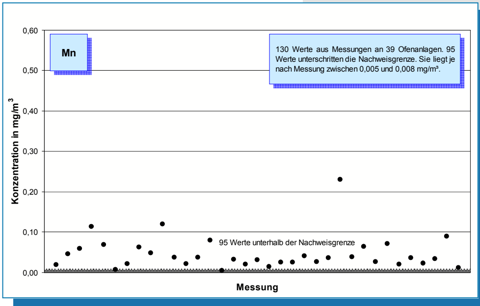
Bild 5-43: Messwerte (Jahr 2006) der Mangan-Konzentration im Reingas von 39 Drehofenanlagen.
