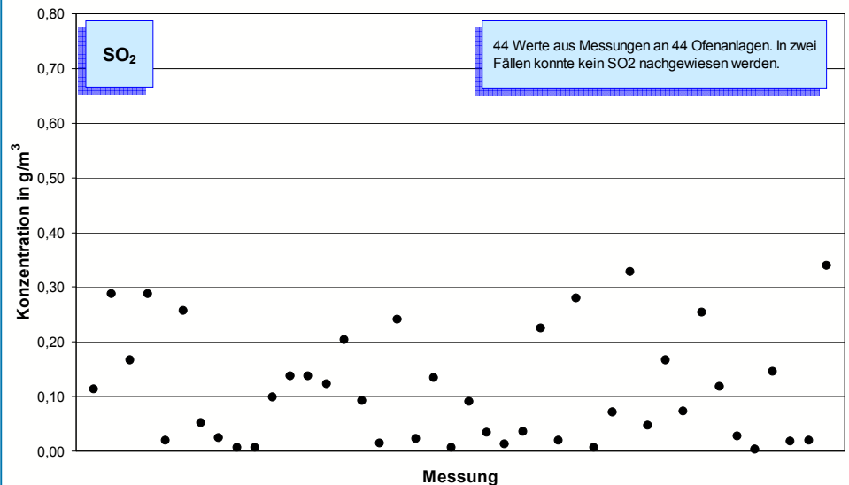
Bild 5-5: Mittelwerte (Jahr 2006) der SO 2 -Konzentration im Reingas von 44 Drehofenanlagen. In zwei Fällen konnte kein SO 2 nachgewiesen werden.
