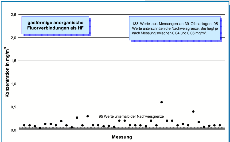
Bild 5-23: Messwerte (Jahr 2006) der Konzentration gasförmiger anorganischer Fluorverbindungen, berechnet als HF, im Reingas von 39 Drehhofenanlagen.
