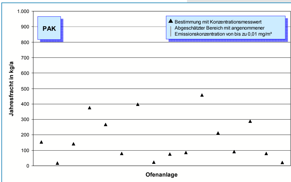
Bild 5-16: PAK-Emissionen (Jahresfracht 2006) von 16 Drehofenanlagen.
