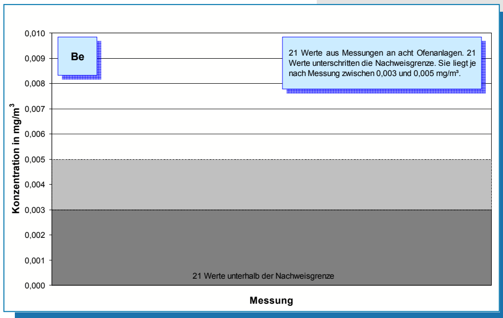
Bild 5-51: Messwerte (Jahr 2006) der Beryllium-Konzentration im Reingas von acht Drehofenanlagen.
