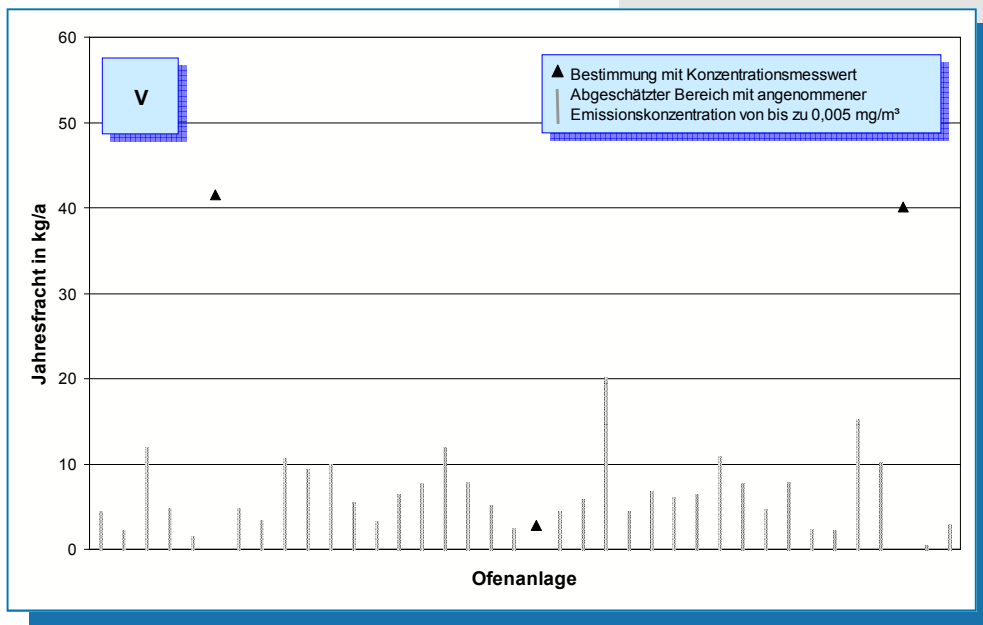
Bild 5-48: Vanadium-Emissionen (Jahresfracht 2006) von 38 Drehofenanlagen.
