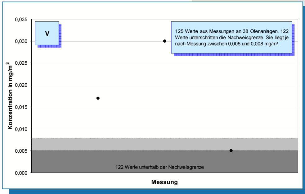
Bild 5-47: Messwerte (Jahr 2006) der Vanadium-Konzentration im Reingas von 38 Drehofenanlagen.
