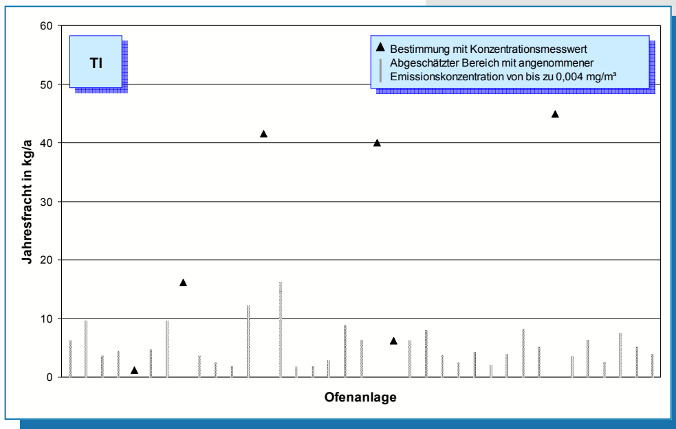
Bild 5-28: Thallium-Emissionen (Jahresfracht 2006) von 37 Drehofenanlagen.
