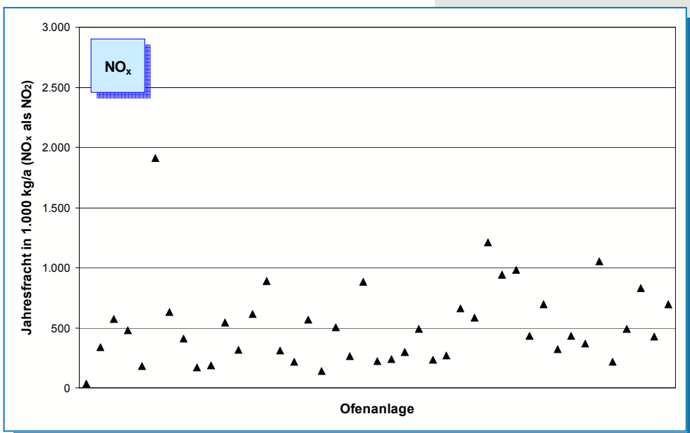
Bild 5-4: NO x -Emissionen (Jahresfracht 2006) von 43 Drehofenanlagen.
