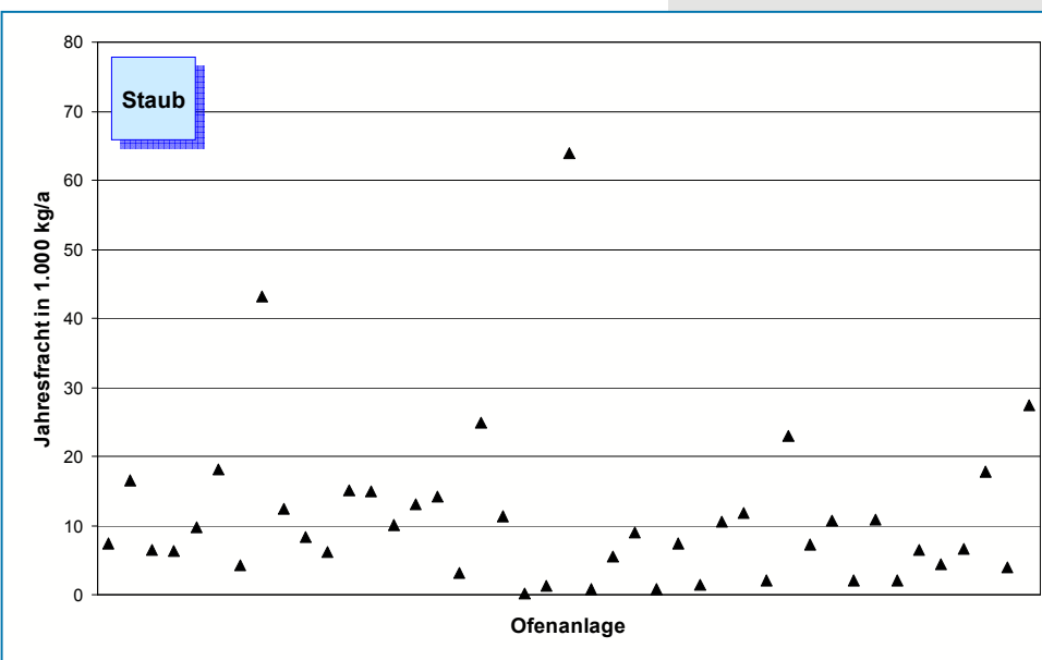
Bild 5-2: Staub-Emissionen (Jahresfracht 2006) von 43 Drehofenanlagen.
