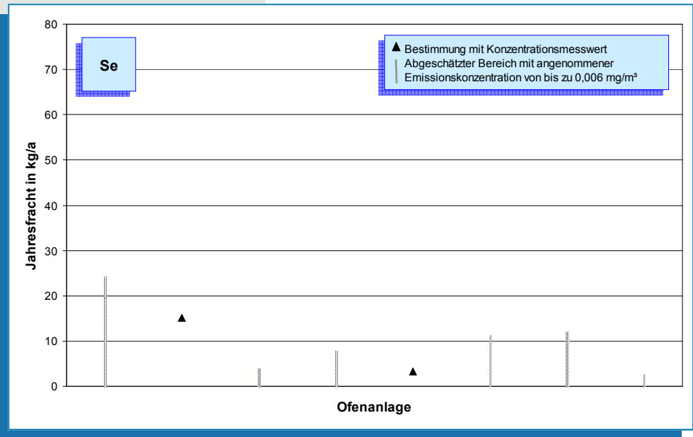
Bild 5-54: Selen-Emissionen (Jahresfracht 2006) von acht Drehofenanlagen. Bei Messungen unterhalb der Nachweisgrenze kann die Fracht nur abgeschätzt werden. Der Bereich möglicher Emissionen ist in diesen Fällen als Linie dargestellt, deren Obergrenze mit einer Konzentration von 0,006 mg/m 3 berechnet wurde.
