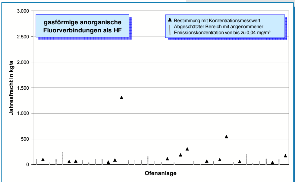
Bild 5-24: HF-Emissionen (Jahresfracht 2006) von 39 Drehhofenanlagen.
