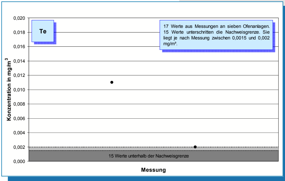
Bild 5-55: Messwerte (Jahr 2006) der Tellur-Konzentration im Reingas von sieben Drehofenanlagen.
