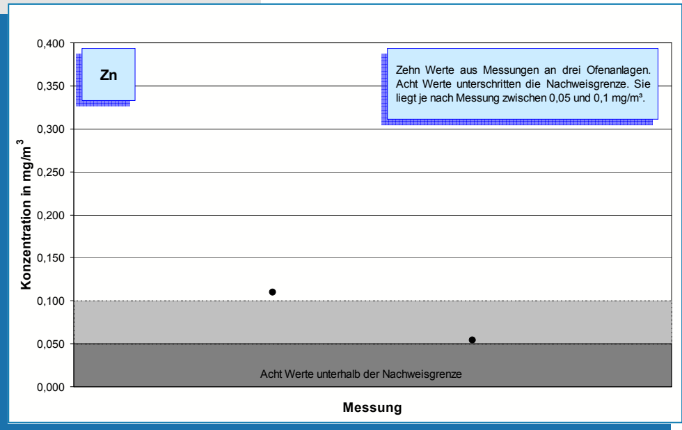
Bild 5-57: Messwerte (Jahr 2006) der Zink-Konzentration im Reingas von drei Drehofenanlagen.
