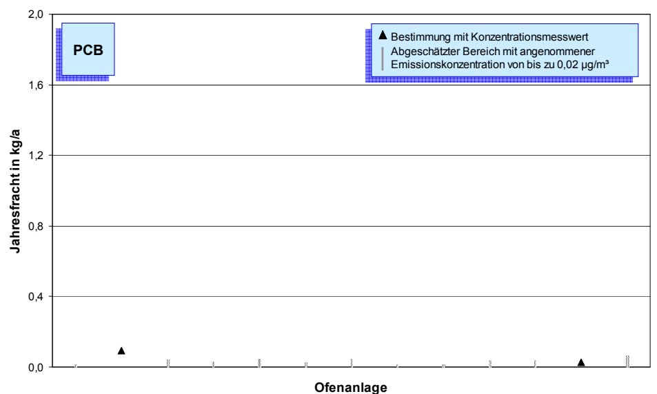
Bild 5-14: PCB-Emissionen (Jahresfracht 2006) von 13 Drehofenanlagen.
