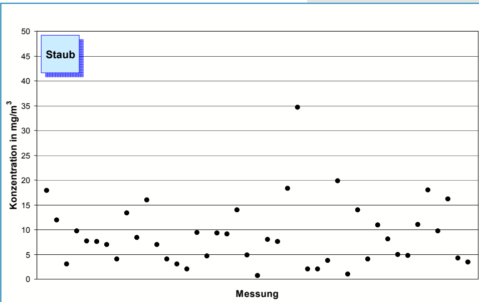
Bild 5-1: Mittelwerte (Jahr 2006) der Staubkonzentration im Reingas von 43 Drehofenanlagen.
