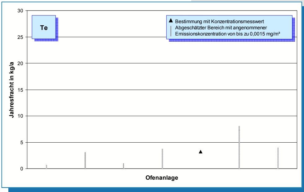
Bild 5-56: Tellur-Emissionen (Jahresfracht 2006) von sieben Drehofenanlagen.
