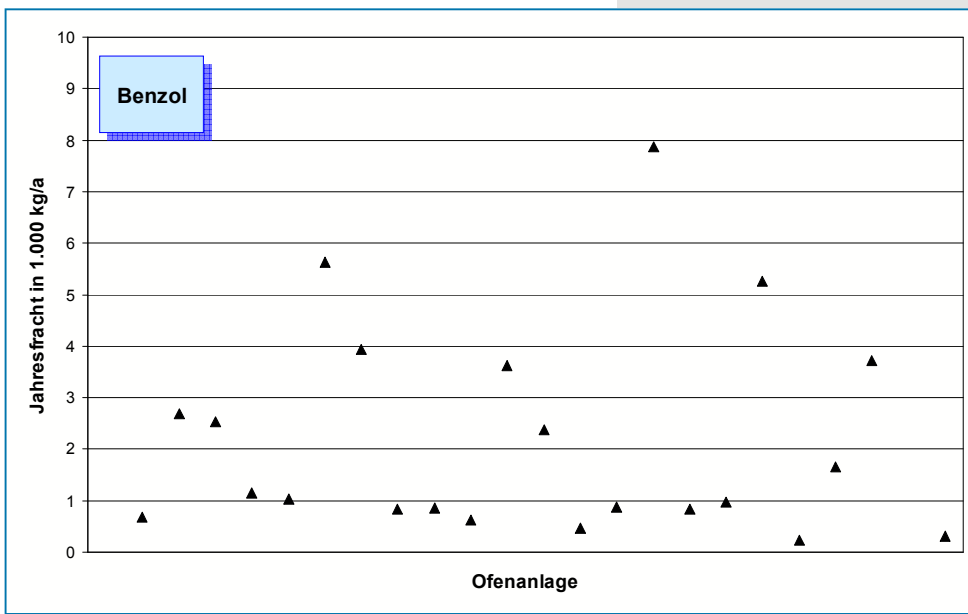
Bild 5-20: Benzol-Emissionen (Jahresfracht 2006) von 22 Drehofenanlagen.
