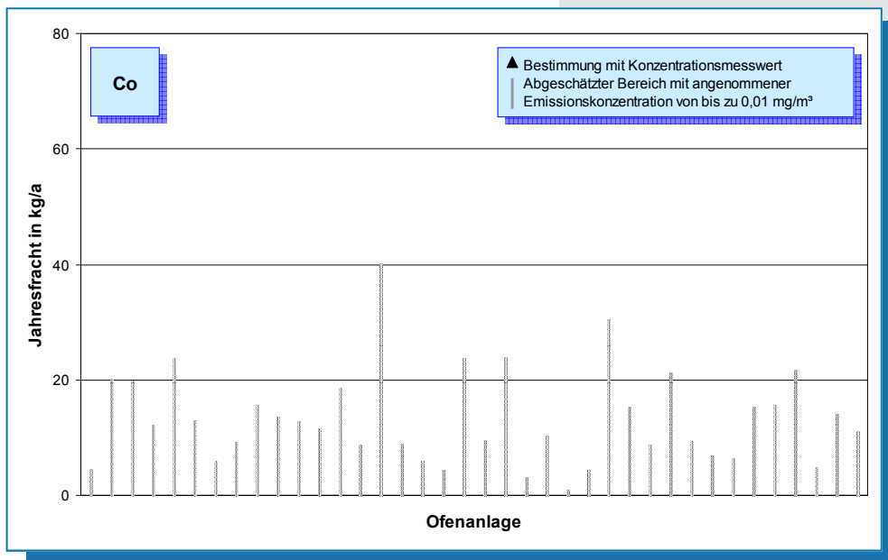
Bild 5-40: Cobalt-Emissionen (Jahresfracht 2006) von 39 Drehofenanlagen.
