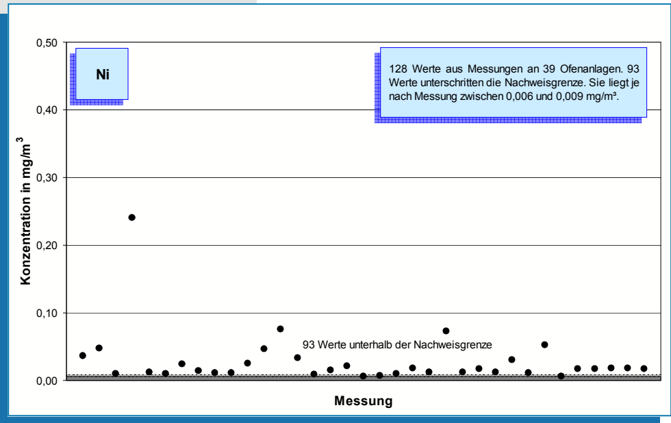
Bild 5-45: Messwerte (Jahr 2006) der Nickel-Konzentration im Reingas von 39 Drehofenanlagen.
