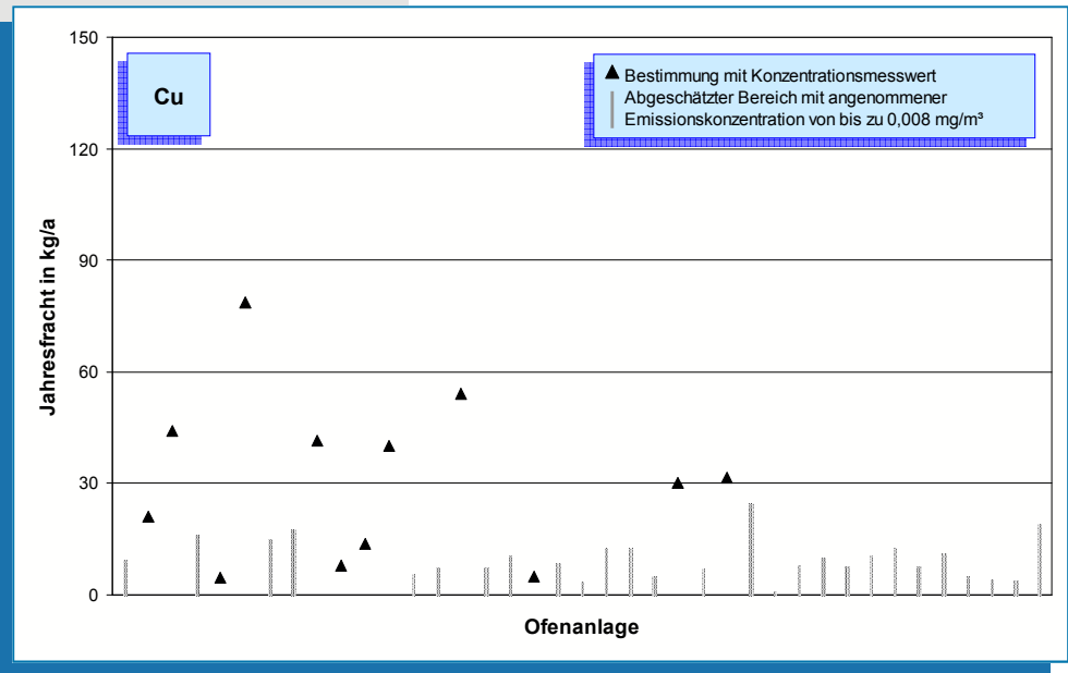
Bild 5-42: Kupfer-Emissionen (Jahresfracht 2006) von 39 Drehofenanlagen. Bei Messungen unterhalb der Nachweisgrenze kann die Fracht nur abgeschätzt werden. Der Bereich möglicher Emissionen ist in diesen Fällen als Linie dargestellt, deren Obergrenze mit einer Konzentration von 0,008 mg/m 3 berechnet wurde.
