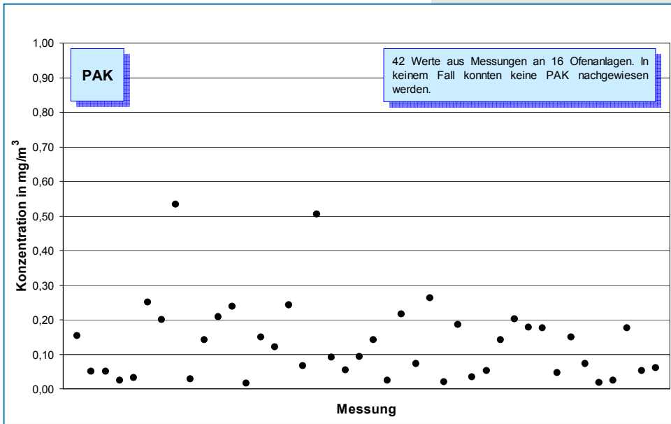
Bild 5-15: Messwerte (Jahr 2006) der Konzentration von polycyclischen aromatischen Kohlenwasserstoffen (PAK nach EPA 610) im Reingas von 16 Drehofenanlagen. In keinem Fall konnten keine PAK nachgewiesen werden. Eine Nachweisgrenze lässt sich aus der Norm nicht ableiten. Bei den derzeit eingesetzten Messverfahren sind gemessene Emissionskonzentrationen unterhalb von 0,1 \text{ mg}/\text{m}^3 nicht abgesichert.
