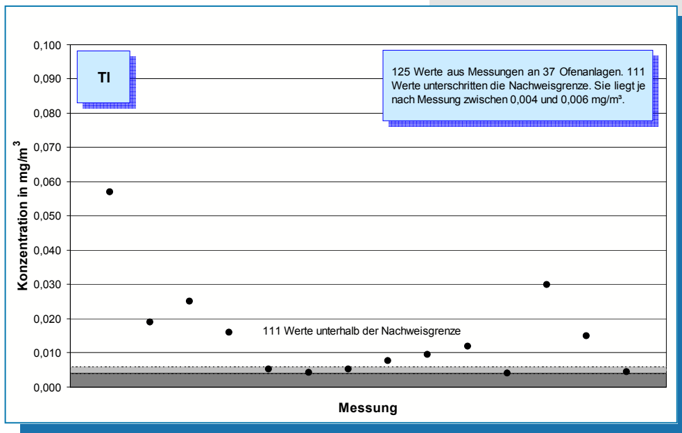
Bild 5-27: Messwerte (Jahr 2006) der Thallium-Konzentration im Reingas von 37 Drehofenanlagen.
