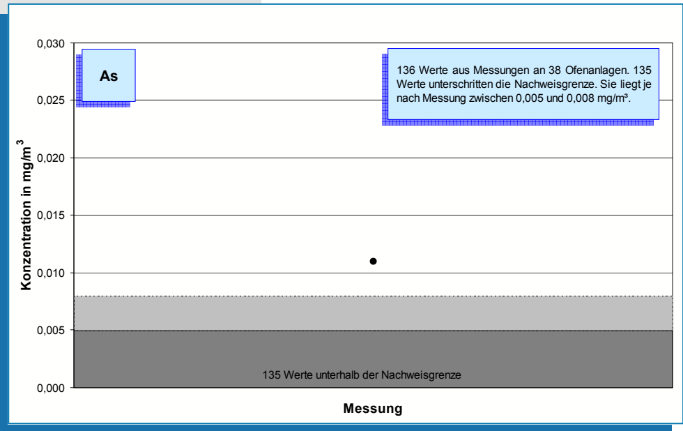
Bild 5-33: Messwerte (Jahr 2006) der Arsen-Konzentration im Reingas von 38 Drehofenanlagen.
