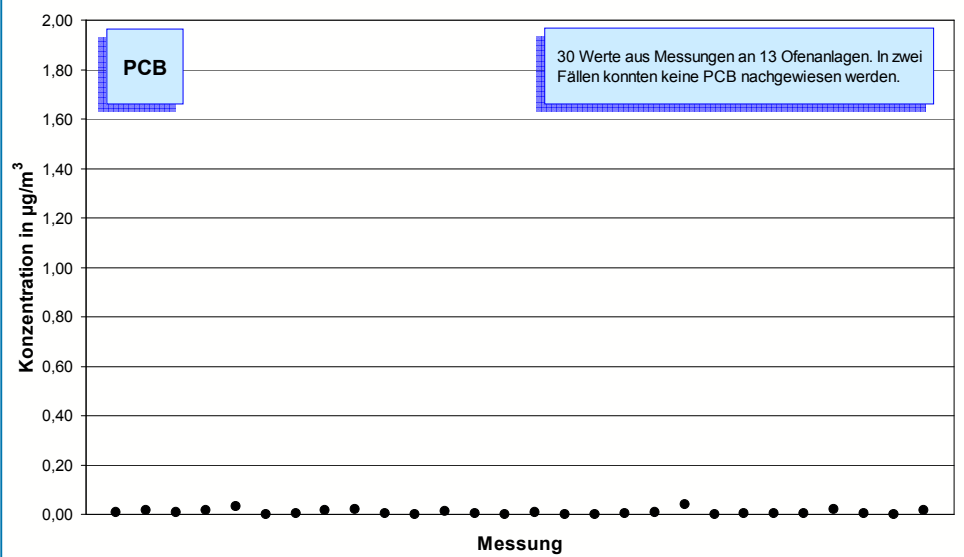
Bild 5-13: Messwerte (Jahr 2006) der Konzentration von polychlorierten Biphenylen (PCB nach DIN 51527) im Reingas von 13 Drehofenanlagen. In zwei Fällen konnten keine PCB nachgewiesen werden.
