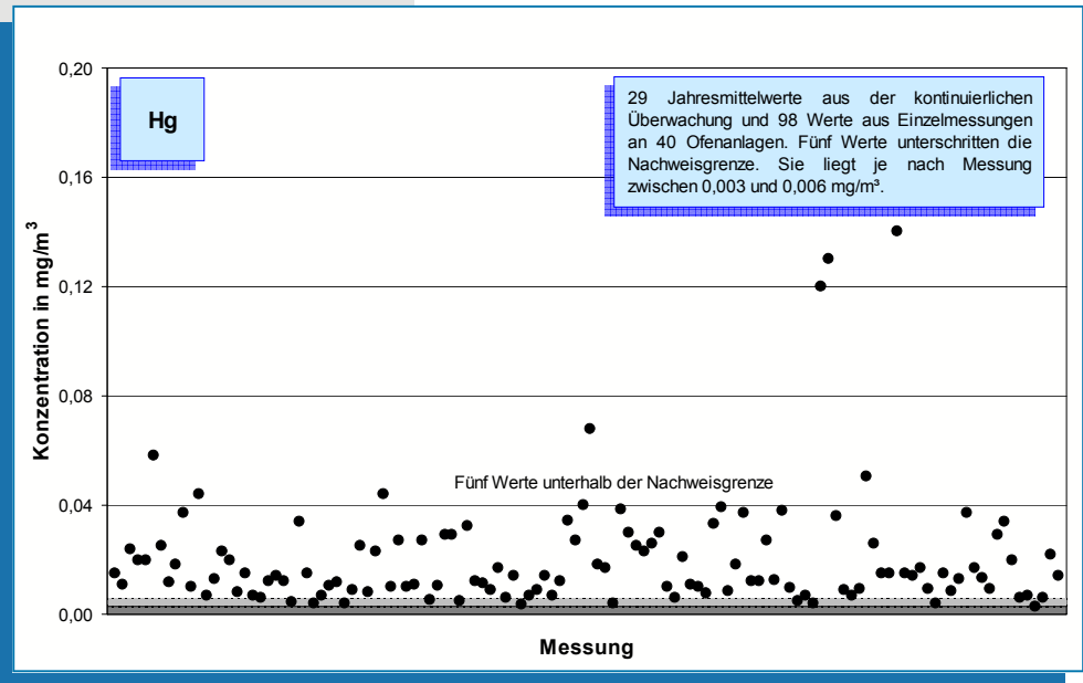
Bild 5-29: Messwerte (Jahr 2006) der Quecksilber-Konzentration im Reingas von 40 Drehofenanlagen.
