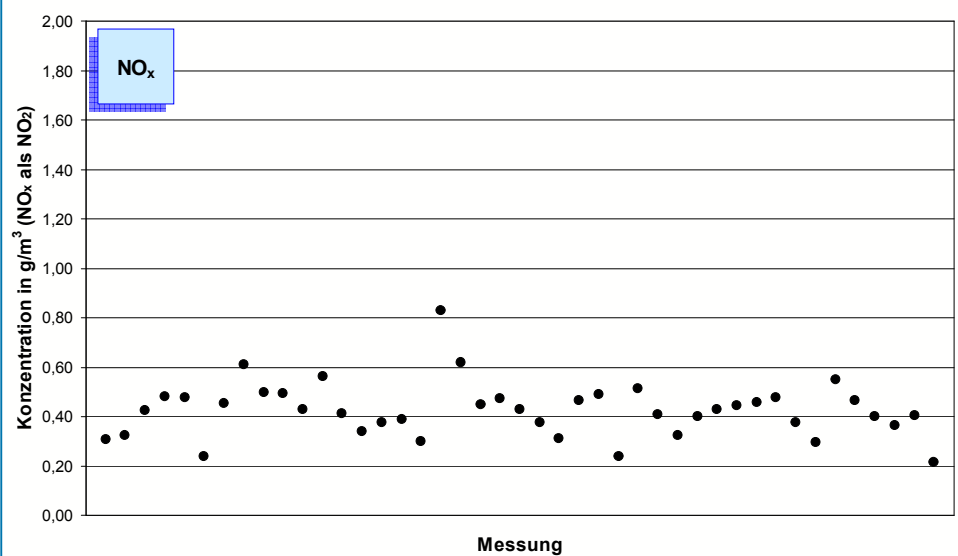
Bild 5-3: Mittelwerte (Jahr 2006) der NO x -Konzentration im Reingas von 43 Drehofenanlagen. Anmerkung: im Jahr 2006 überstiegen die Emissionen mehrerer Anlagen die heute in der TA Luft für Zementwerke vorgesehenen Emissionswerte. Die Betriebsgenehmigungen für diese Werke beruhen noch auf höheren NO x -Grenzwerten. Einige dieser Anlagen wurden inzwischen bzw. werden derzeit mit einer Anlage zur NO x -Minderung nachgerüstet.
