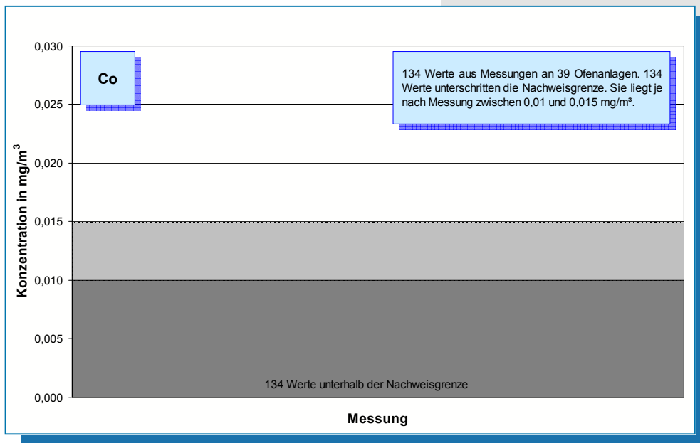
Bild 5-39: Messwerte (Jahr 2006) der Cobalt-Konzentration im Reingas von 39 Drehofenanlagen.
