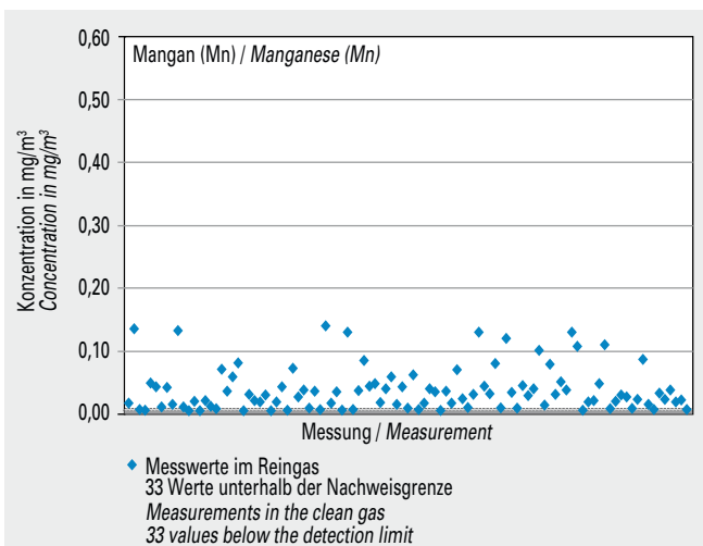
Bild 5-43 Messwerte (Jahr 2013) der Konzentration von Mangan (Mn) im Reingas von 38 Drehofenanlagen.
