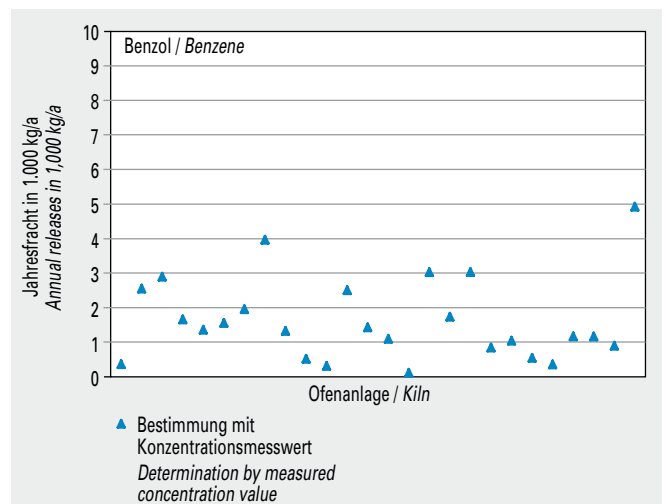
Bild 5-20 Emissionen von Benzol (Jahresfracht 2013) von 26 Drehofenanlagen. Fig. 5-20 Benzene emissions (annual releases in 2013) of 26 rotary kilns.
