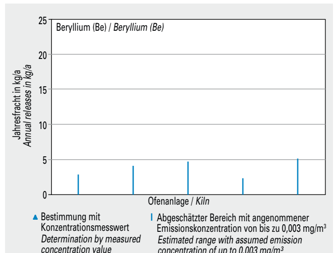
Bild 5-52 Emissionen von Beryllium (Be) von fünf Drehofenanlagen (Jahresfracht 2013).
