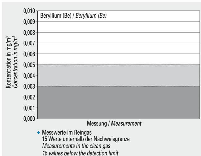
Bild 5-51 Messwerte (Jahr 2013) der Konzentration von Beryllium (Be) im Reingas von fünf Drehofenanlagen.
