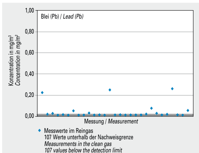
Bild 5-35 Messwerte (Jahr 2013) der Konzentration von Blei (Pb) im Reingas von 38 Drehofenanlagen.
