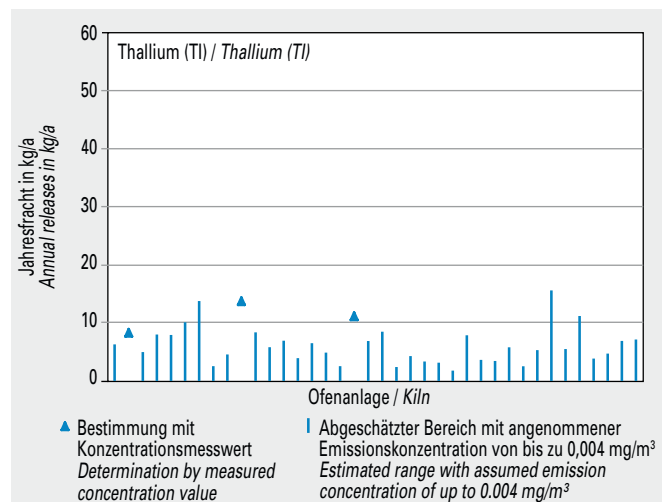
Bild 5-28 Emissionen von Thallium (Tl) von 38 Drehofenanlagen (Jahresfracht 2013).
