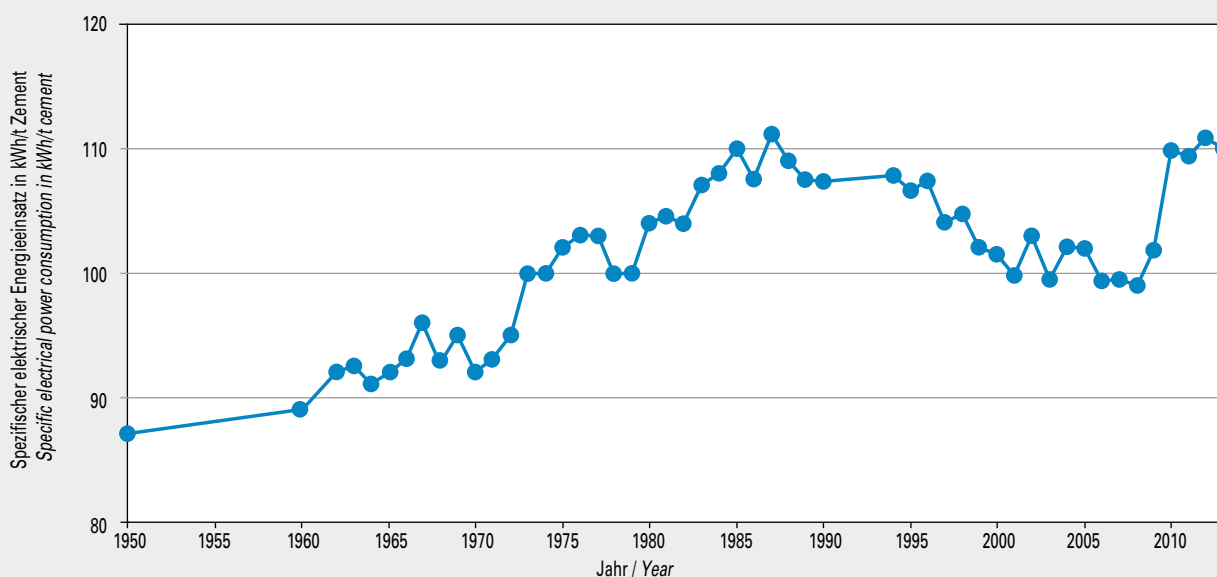
Bild 4-2 Entwicklung des spezifischen elektrischen Energieeinsatzes (Berücksichtigung der neuen Bundesländer seit 1987) [2]. Fig. 4-2 Development of the specific electrical power demand (New Federal States included since 1987) [2].
