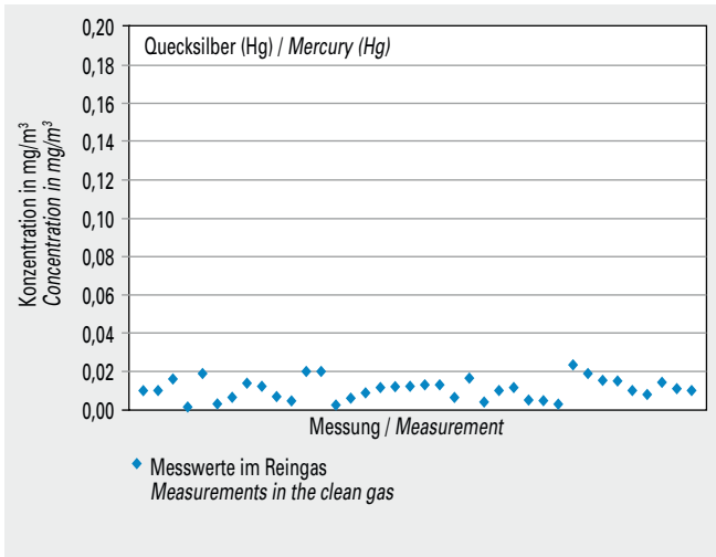
Bild 5-29 Mittelwerte (Jahr 2013) der Konzentration von Quecksilber (Hg) im Reingas von 38 Drehofenanlagen. Fig. 5-29 Mercury (Hg) concentration values (year 2013) measured in the clean gas of 38 rotary kilns.
