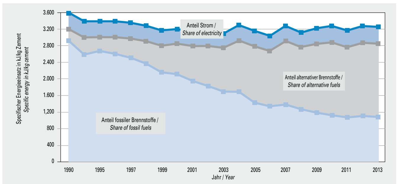
Bild 4-1 Entwicklung des spezifischen Energieeinsatzes [2]. Fig. 4-1 Development of the specific fuel energy demand [2].
