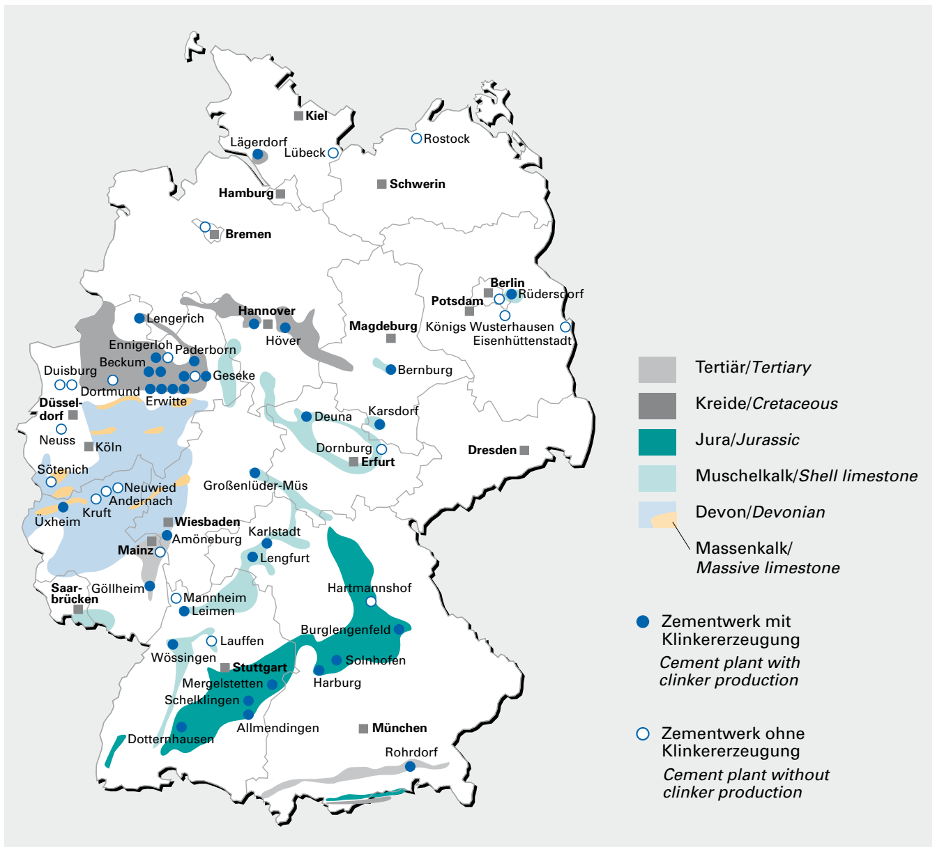
Bild 2-1 Zementwerke in der Bundesrepublik Deutschland im Jahr 2014. Fig. 2-1 Cement works in the Federal Republic of Germany in the year 2014.
