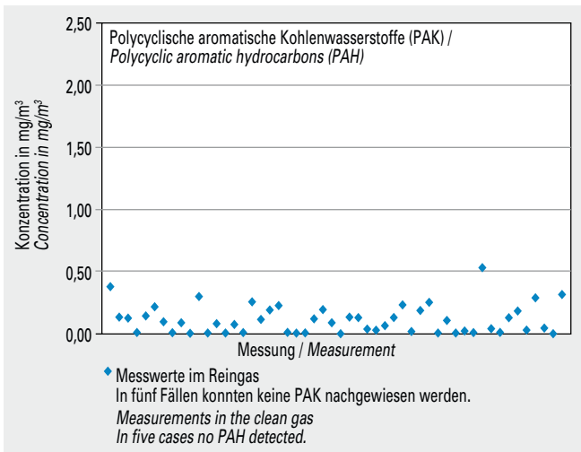
Bild 5-15 Messwerte (Jahr 2013) der Konzentration von PAK (nach EPA 610) im Reingas von 16 Drehofenanlagen.
