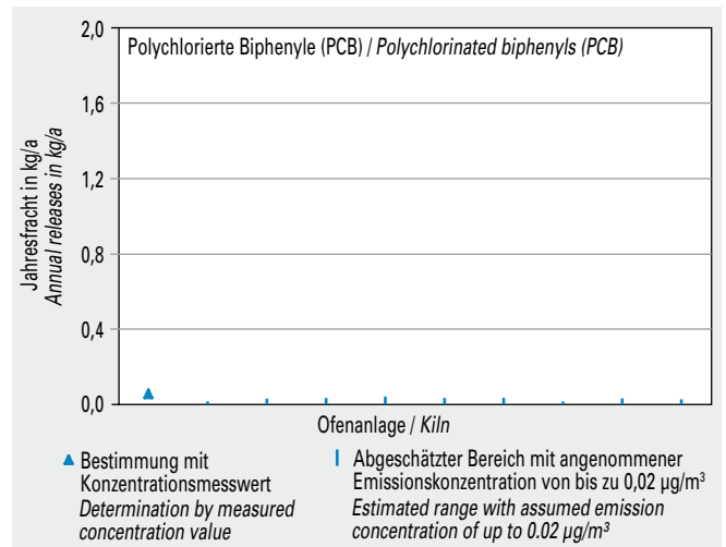
Bild 5-14 Emissionen von polychlorierten Biphenylen (PCB) von zehn Drehofenanlagen (Jahresfracht 2013). Fig. 5-14 Polychlorinated biphenyl (PCB) emissions (annual releases in 2013) of ten rotary kilns.
