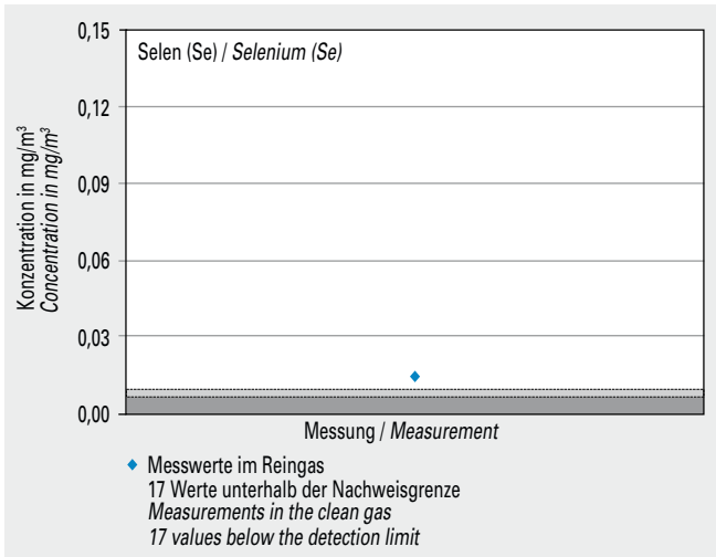
Bild 5-53 Messwerte (Jahr 2013) der Konzentration von Selen (Se) im Reingas von sechs Drehofenanlagen.
