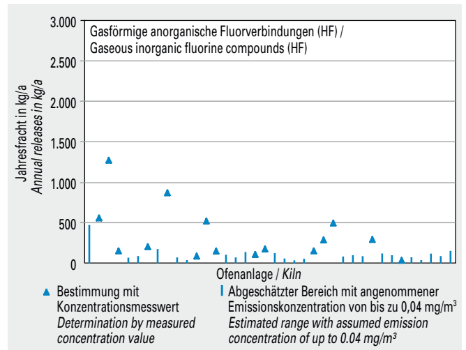
Bild 5-24 Emissionen von gasförmigen anorganischen Fluorverbindungen (HF) von 38 Drehofenanlagen (Jahresfracht 2013). Fig. 5-24 Gaseous inorganic fluorine compounds (HF) emissions (annual releases in 2013) of 38 rotary kilns.
