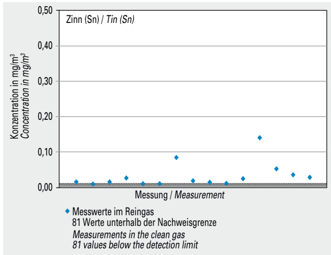
Bild 5-49 Messwerte (Jahr 2013) der Konzentration von Zinn (Sn) im Reingas von 27 Drehofenanlagen.
