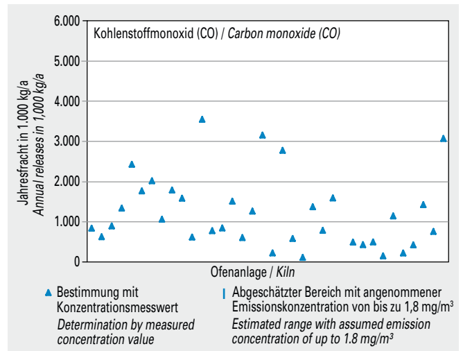
Bild 5-8 Emissionen von Kohlenstoffmonoxid (CO) von 36 Drehofenanlagen (Jahresfracht 2013).
