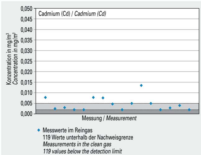
Bild 5-25 Messwerte (Jahr 2013) der Konzentration von Cadmium (Cd) im Reingas von 38 Drehofenanlagen.
