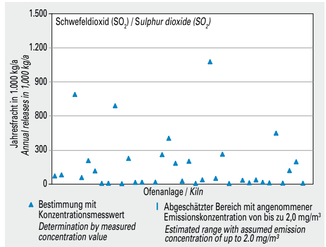
Bild 5-6 Emissionen von Schwefeldioxid (SO 2 ) von 39 Drehofenanlagen (Jahresfracht 2013).
