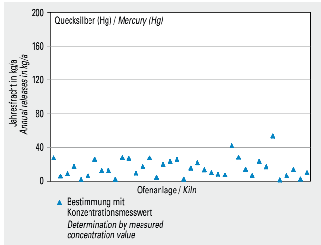
Bild 5-30 Emissionen von Quecksilber (Hg) von 38 Drehofenanlagen (Jahresfracht 2013). Fig. 5-30 Mercury (Hg) emissions (annual releases in 2013) of 38 rotary kilns.
