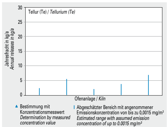
Bild 5-56 Emissionen von Tellur (Te) von fünf Drehofenanlagen (Jahresfracht 2013).
