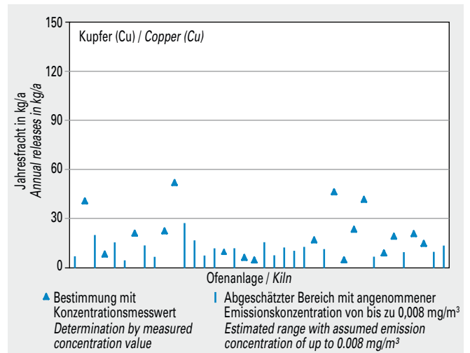
Bild 5-42 Emissionen von Kupfer (Cu) von 38 Drehofenanlagen (Jahresfracht 2013).
