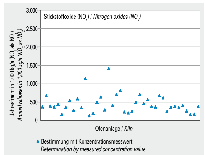
Bild 5-4 Emissionen von Stickstoffoxiden (NO x ) von 41 Drehofenanlagen (Jahresfracht 2013).
