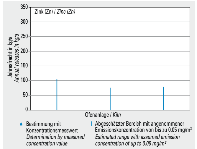
Bild 5-58 Emissionen von Zink (Zn) von drei Drehofenanlagen (Jahresfracht 2013).
