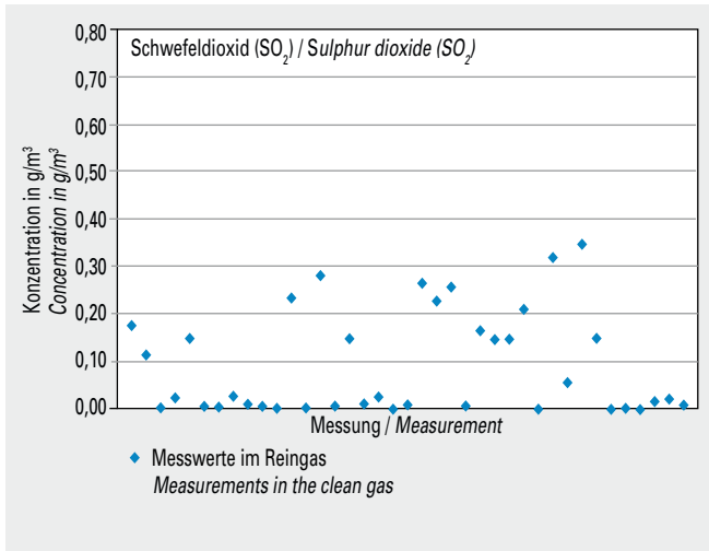
Bild 5-5 Messwerte (Jahr 2013) der Konzentration von Schwefeldioxid (SO 2 ) im Reingas von 39 Drehofenanlagen.
