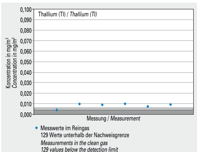
Bild 5-27 Messwerte (Jahr 2013) der Konzentration von Thallium (Tl) im Reingas von 38 Drehofenanlagen.
