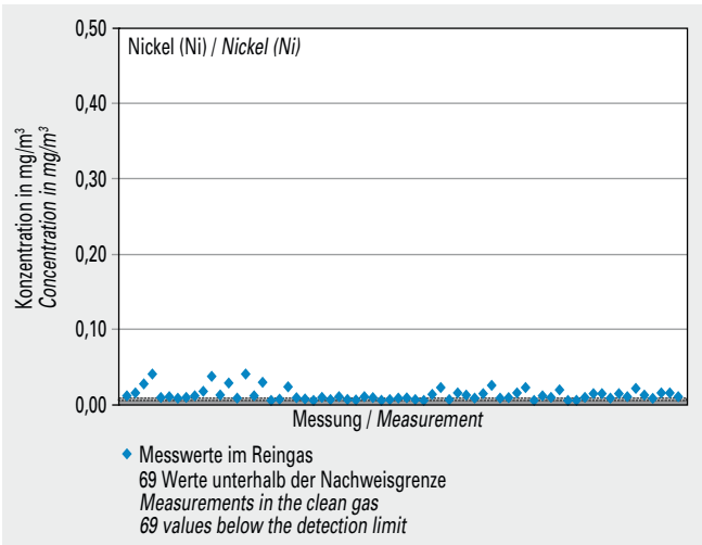
Bild 5-45 Messwerte (Jahr 2013) der Konzentration von Nickel (Ni) im Reingas von 37 Drehofenanlagen.
