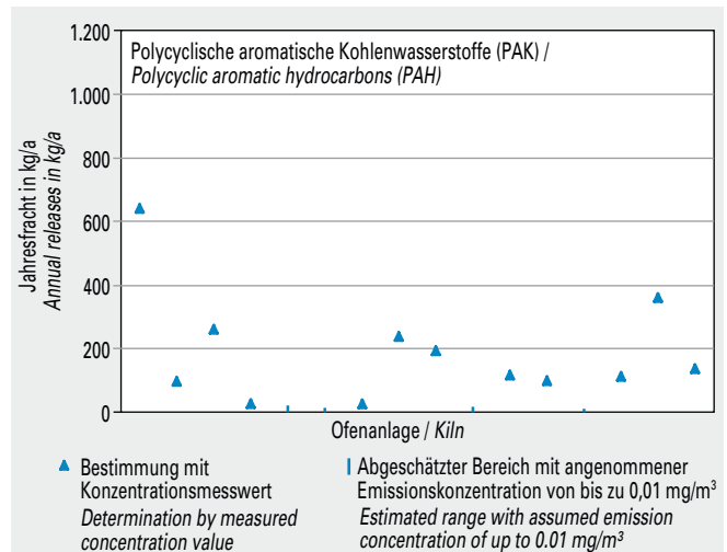
Bild 5-16 Emissionen von polycyclischen aromatischen Kohlenwasserstoffen (PAK) von 16 Drehofenanlagen (Jahresfracht 2013).
