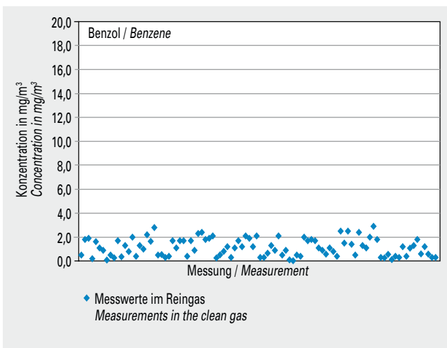
Bild 5-19 Messwerte (Jahr 2013) der Konzentration von Benzol im Reingas von 26 Drehofenanlagen. Fig. 5-19 Benzene concentration values (year 2013) measured in the clean gas of 26 rotary kilns.
