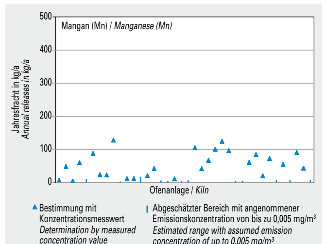
Bild 5-44 Emissionen von Mangan (Mn) von 38 Drehofenanlagen (Jahresfracht 2013).
