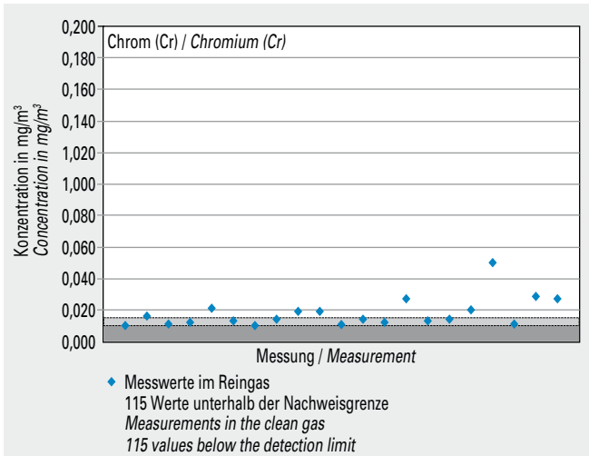
Bild 5-37 Messwerte (Jahr 2013) der Konzentration von Chrom (Cr) im Reingas von 38 Drehofenanlagen.
