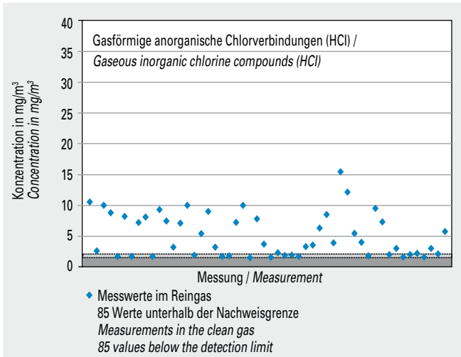
Bild 5-21 Messwerte (Jahr 2013) der Konzentrationen gasförmiger anorg. Chlorverbindungen (HCl) im Reingas von 38 Drehofenanlagen. Fig. 5-21 Gaseous inorganic chlorine compounds (HCl) concentration values (year 2013) measured in the clean gas of 38 rotary kilns.
