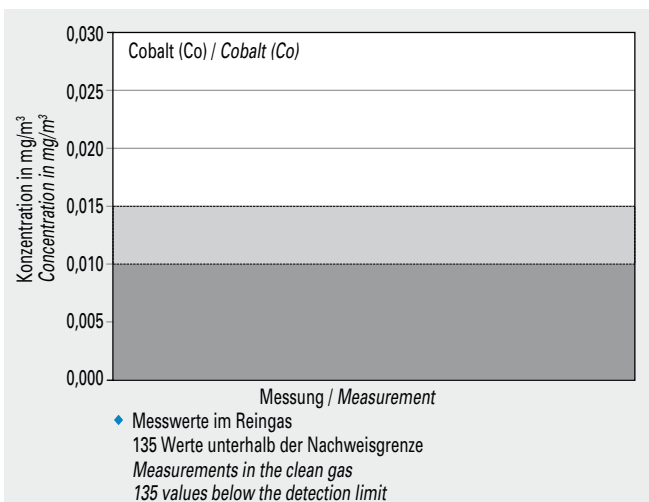
Bild 5-39 Messwerte (Jahr 2013) der Konzentration von Cobalt (Co) im Reingas von 38 Drehofenanlagen.
