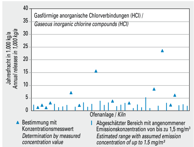
Bild 5-22 Emissionen von gasförmigen anorganischen Chlorverbindungen (HCl) von 38 Drehofenanlagen (Jahresfracht 2013). Fig. 5-22 Gaseous inorganic chlorine compounds (HCl) emissions (annual releases in 2013) of 38 rotary kilns.
