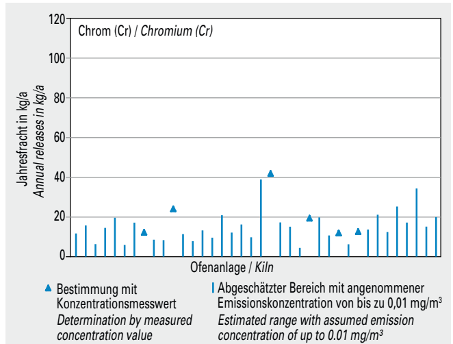
Bild 5-38 Emissionen von Chrom (Cr) von 38 Drehofenanlagen (Jahresfracht 2013).
