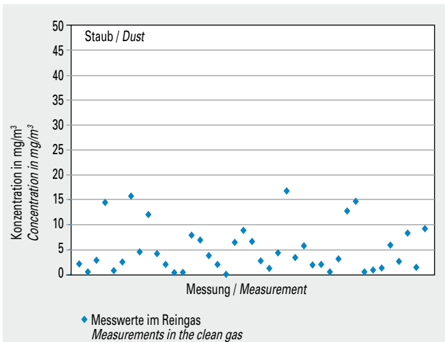
Bild 5-1 Mittelwerte (Jahr 2013) der Konzentration von Staub im Reingas von 41 Drehofenanlagen.
