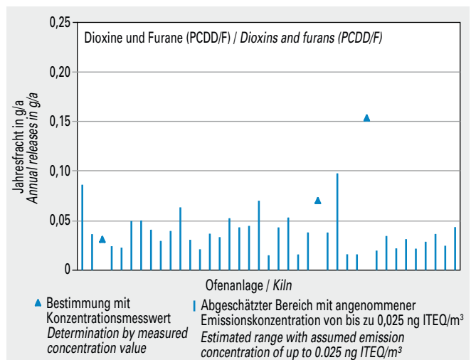
Bild 5-12 Emissionen von Dioxinen und Furanen (PCDD/F) von 39 Drehofenanlagen (Jahresfracht 2013). Fig. 5-12 Dioxin and furan emissions (annual releases in 2013) of 39 rotary kilns.
