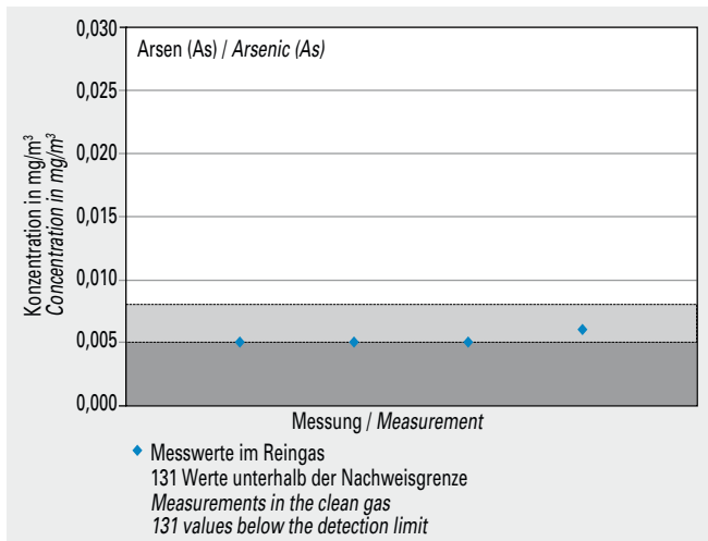
Bild 5-33 Messwerte (Jahr 2013) der Konzentration von Arsen (As) im Reingas von 37 Drehofenanlagen.
