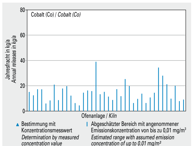
Bild 5-40 Emissionen von Cobalt (Co) von 38 Drehofenanlagen (Jahresfracht 2013).
