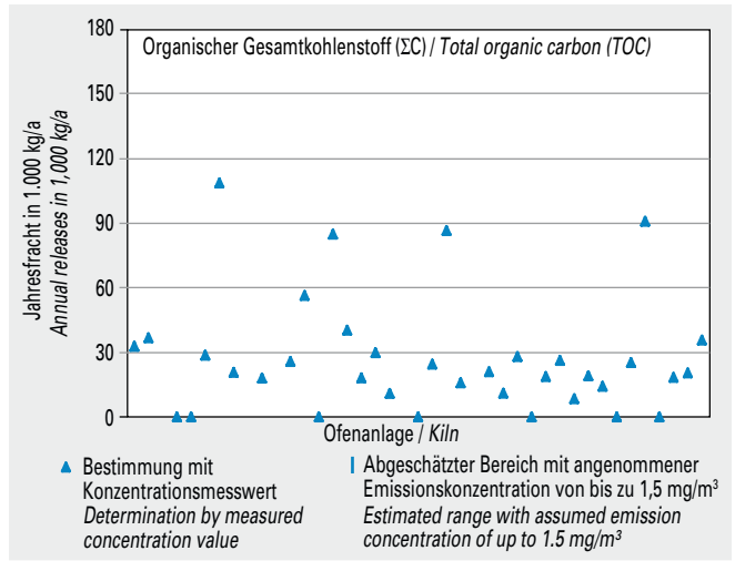
Bild 5-10 Emissionen von organischem Gesamtkohlenstoff (ΣC) von 32 Drehofenanlagen (Jahresfracht 2013). Fig. 5-10 Total organic carbon (TOC) emissions (annual releases in 2013) of 32 rotary kilns.
