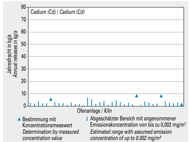
Bild 5-26 Emissionen von Cadmium (Cd) von 38 Drehofenanlagen (Jahresfracht 2013).
