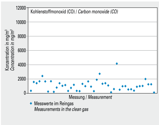
Bild 5-7 Messwerte (Jahr 2013) der Konzentration von Kohlenstoffmonoxid (CO) im Reingas von 36 Drehofenanlagen.
