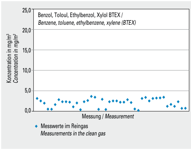
Bild 5-17 Messwerte (2013) der Konzentration von Benzol, Toluol, Ethylbenzol und Xylol (BTEX) im Reingas von 11 Drehofenanlagen. Fig. 5-17 Benzene, Toluene, ethylbenzene, xylene (BTEX) concentration values (year 2013) measured in the clean gas of 11 rotary kilns.
