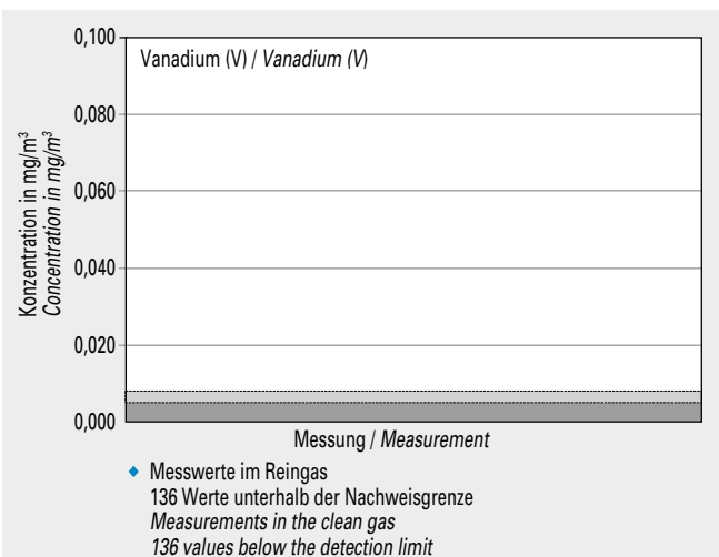
Bild 5-47 Messwerte (Jahr 2013) der Konzentration von Vanadium (V) im Reingas von 38 Drehofenanlagen.
