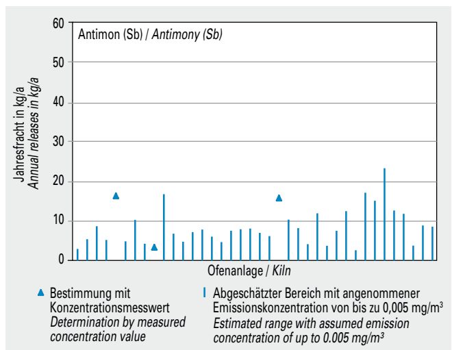
Bild 5-32 Emissionen von Antimon (Sb) von 38 Drehofenanlagen (Jahresfracht 2013). Fig. 5-32 Antimony (Sb) emissions (annual releases in 2013) of 38 rotary kilns.
