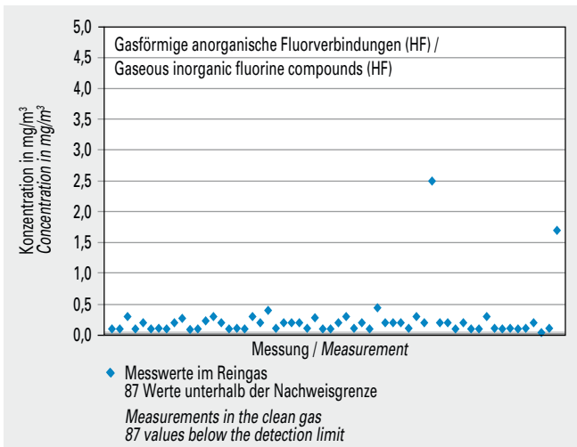
Bild 5-23 Messwerte (Jahr 2013) der Konzentration gasförm. anorg. Fluorverbindungen (HF) im Reingas von 38 Drehofenanlagen. Fig. 5-23 Gaseous inorganic fluorine compounds (HF) concentration values (year 2013) measured in the clean gas of 38 rotary kilns.
