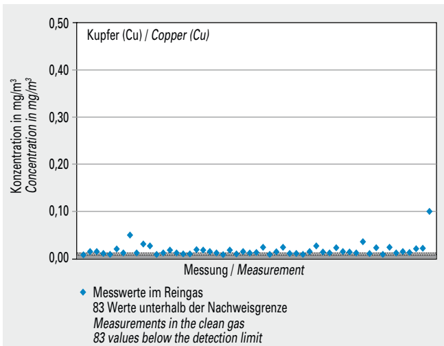
Bild 5-41 Messwerte (Jahr 2013) der Konzentration von Kupfer (Cu) im Reingas von 38 Drehofenanlagen.
