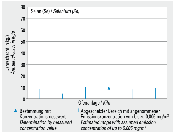
Bild 5-54 Emissionen von Selen (Se) von sechs Drehofenanlagen (Jahresfracht 2013).
