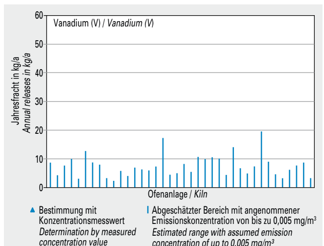
Bild 5-48 Emissionen von Vanadium (V) von 38 Drehofenanlagen (Jahresfracht 2013).
