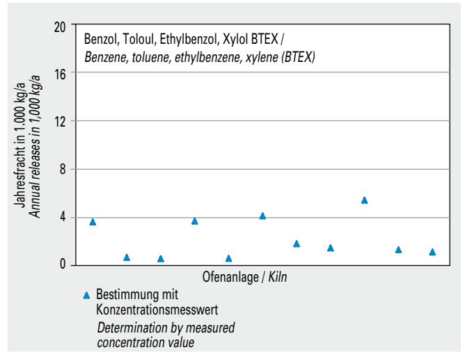
Bild 5-18 Emissionen von Benzol, Toluol, Ethylbenzol, Xylol (BTEX) von 11 Drehofenanlagen (Jahresfracht 2013). Fig. 5-18 Benzene, Toluene, ethylbenzene, xylene (BTEX) emissions (annual releases in 2013) of 11 rotary kilns.
