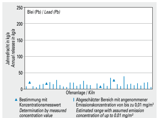
Bild 5-36 Emissionen von Blei (Pb) von 38 Drehofenanlagen (Jahresfracht 2013).
