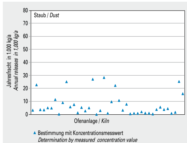
Bild 5-2 Emissionen von Staub (Jahresfracht 2013) von 41 Drehofenanlagen.
