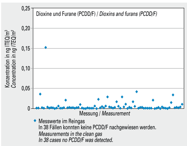
Bild 5-11 Messwerte (Jahr 2013) der Konzentration von Dioxinen und Furanen (PCDD/F) im Reingas von 39 Drehofenanlagen. Fig. 5-11 Dioxin and furan (PCDD/F) concentration values (year 2013) measured in the clean gas of 39 rotary kilns.
