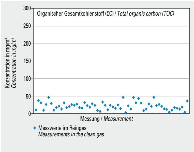
Bild 5-9 Messwerte (Jahr 2013) der Konzentration von organischem Gesamtkohlenstoff (ΣC) im Reingas von 32 Drehofenanlagen. Fig. 5-9 Total organic carbon (TOC) concentration values (year 2013) measured in the clean gas of 32 rotary kilns.
