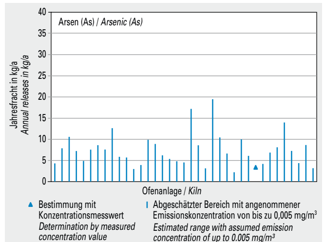
Bild 5-34 Emissionen von Arsen (As) von 37 Drehofenanlagen (Jahresfracht 2013).
