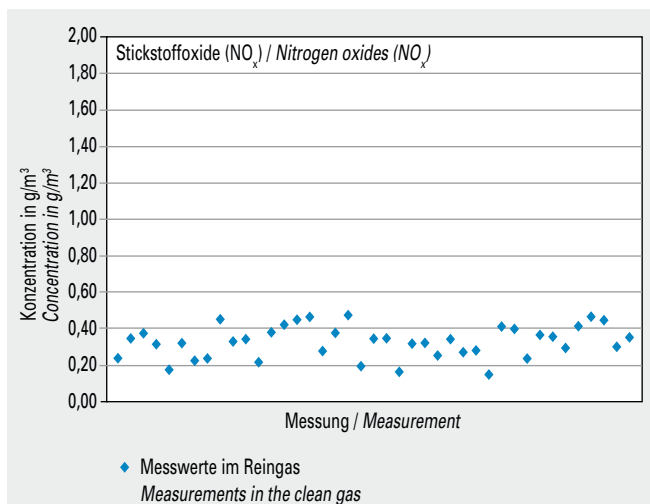
Bild 5-3 Mittelwerte (Jahr 2013) der Konzentration von Stickstoffoxiden (NO x ) im Reingas von 41 Drehofenanlagen.
