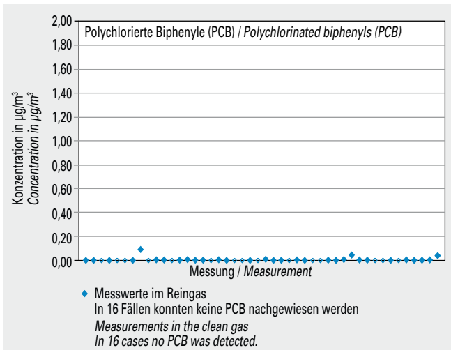
Bild 5-13 Messwerte (Jahr 2013) der Konzentration von polychlorierten Biphenylen (PCB) im Reingas von zehn Drehofenanlagen. Fig. 5-13 Polychlorinated biphenyl (PCB) concentration values (year 2013) measured in the clean gas of ten rotary kilns.
