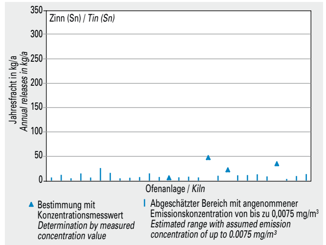
Bild 5-50 Emissionen von Zinn (Sn) von 27 Drehofenanlagen (Jahresfracht 2013).
