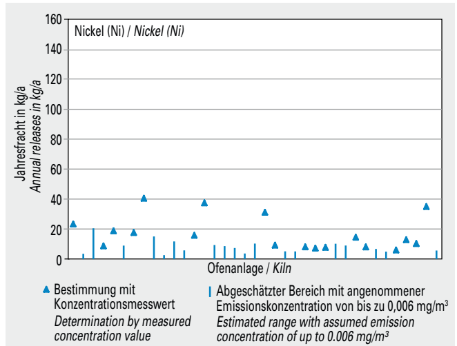
Bild 5-46 Emissionen von Nickel (Ni) von 37 Drehofenanlagen (Jahresfracht 2013).
