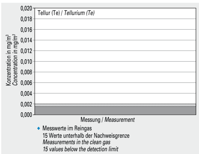
Bild 5-55 Messwerte (Jahr 2013) der Konzentration von Tellur (Te) im Reingas von fünf Drehofenanlagen.
