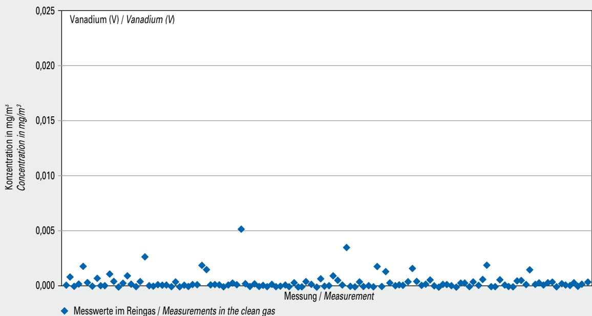
Bild 5-27 Messwerte (Jahr 2019) der Konzentration von Vanadium (V) im Reingas von 36 Drehofenanlagen Fig. 5-27 Vanadium (V) concentration values (year 2019) in the clean gas of 36 rotary kilns
