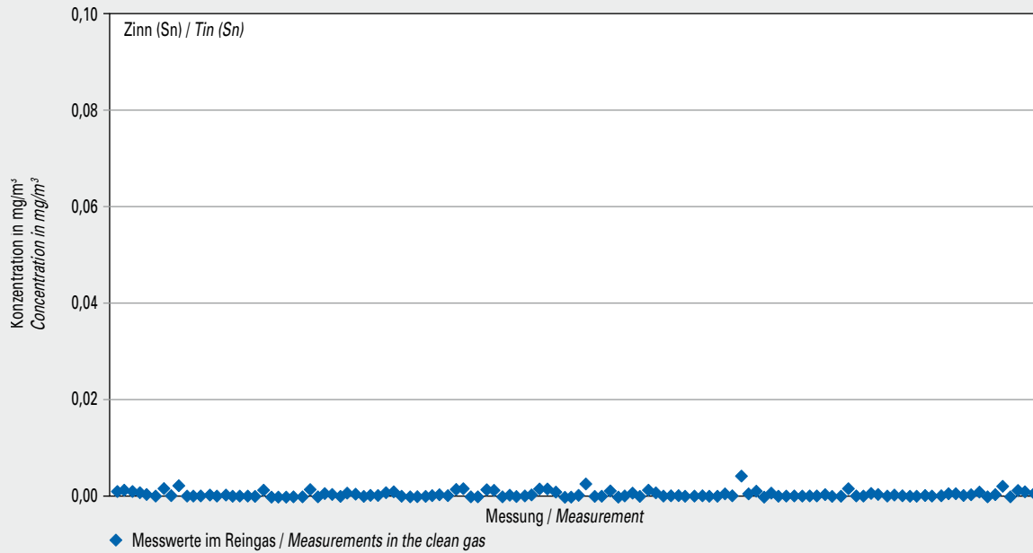
Bild 5-28 Messwerte (Jahr 2019) der Konzentration von Zinn (Sn) im Reingas von 36 Drehofenanlagen Fig. 5-28 Tin (Sn) concentration values (year 2019) in the clean gas of 36 rotary kilns
