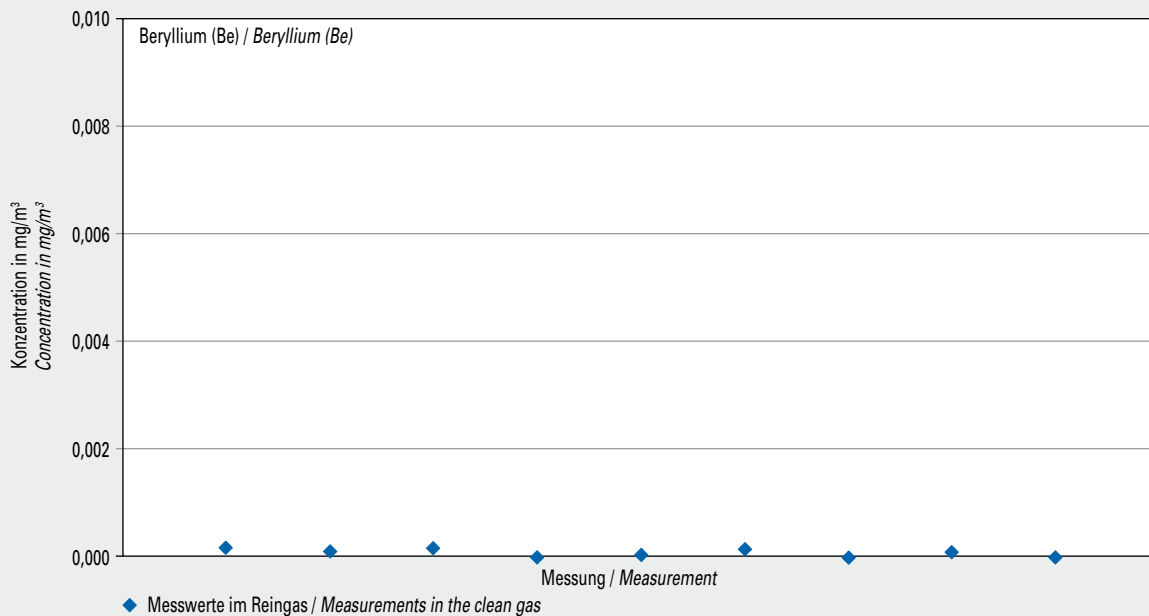
Bild 5-29 Messwerte (Jahr 2019) der Konzentration von Beryllium (Be) im Reingas von drei Drehofenanlagen Fig. 5-29 Beryllium (Be) concentration values (year 2019) in the clean gas of three rotary kilns
